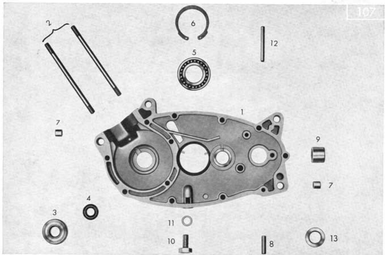
Tafel 13/1 Gehäusehälfte rechts
