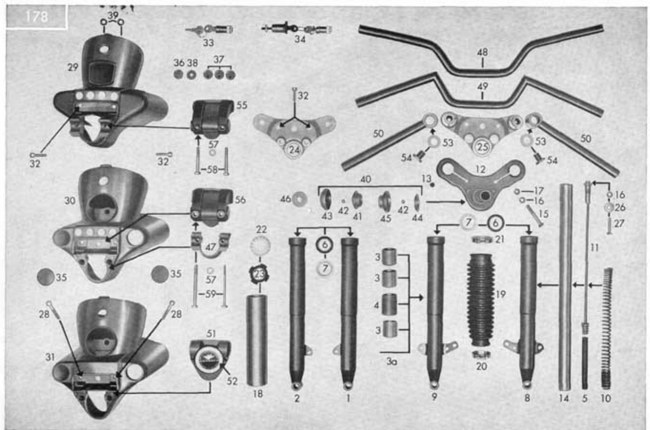
Tafel 27/4 Vorderradgabel, Gabelgehäuse, Lenkungslager, Lenker
