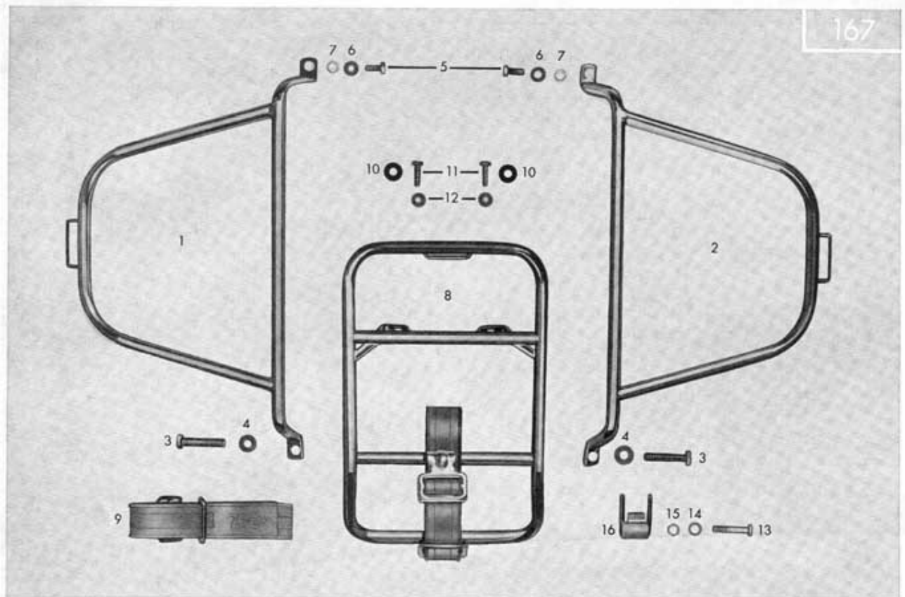
Tafel 39/1 Packtaschenträger, Kofferträger
