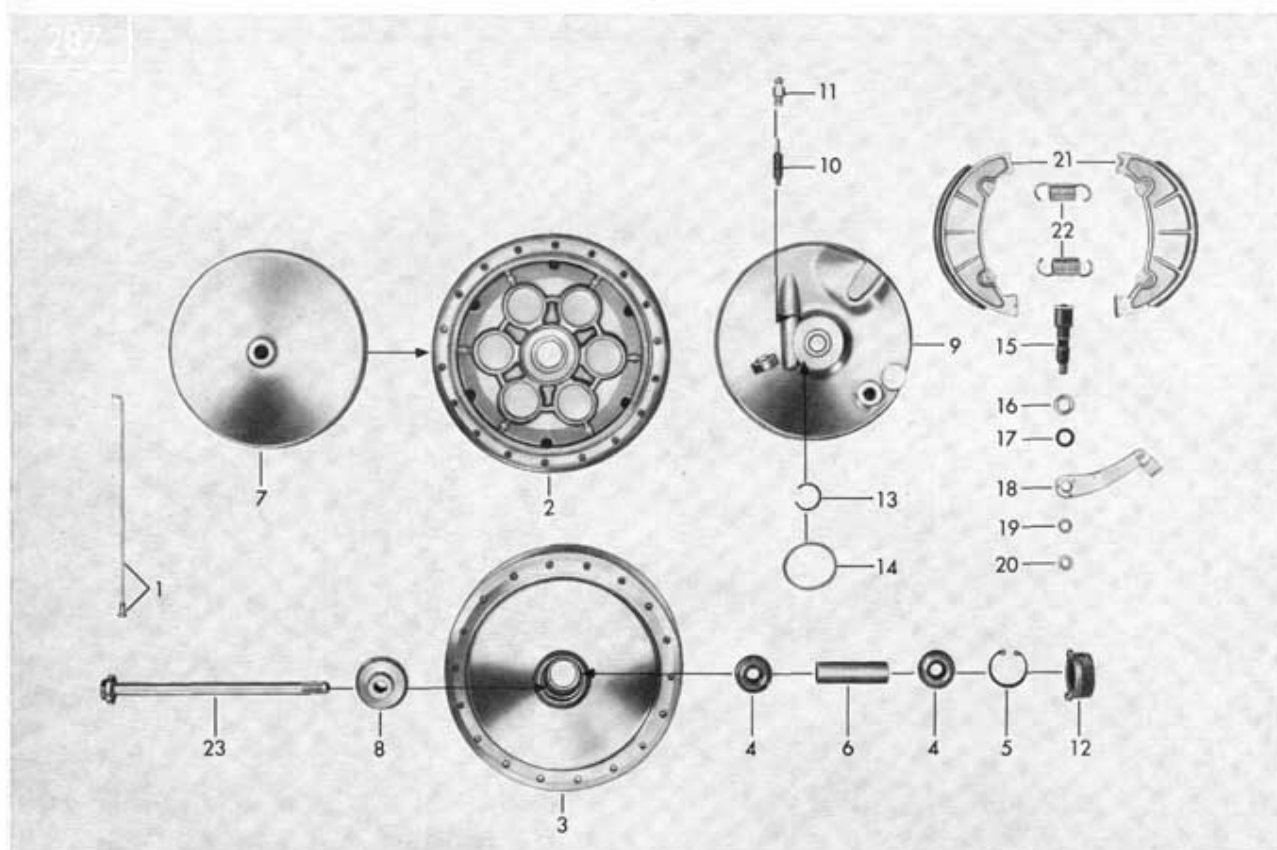
Tafel 30/1 Vorderes Laufrad, Vorderradnabe 150 mm \phi
