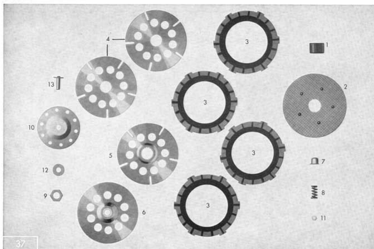
Tafel 22/1 Kupplung
