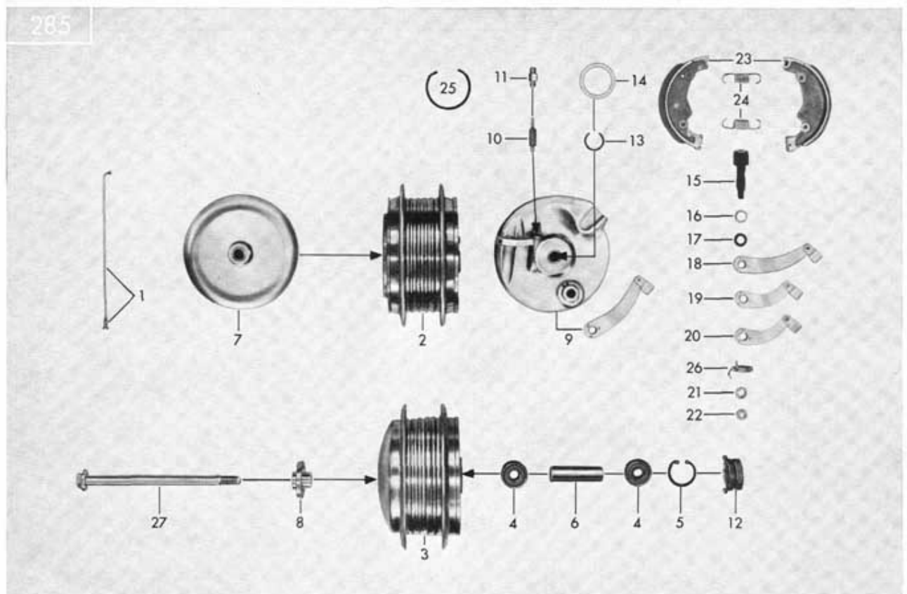
Tafel 29/2 Vorderes Laufrad, Vorderradnabe 120 mm \phi
