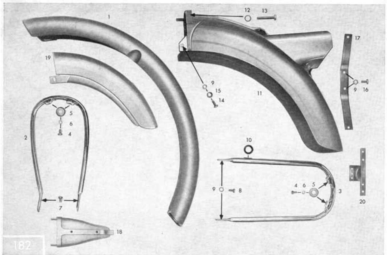
Tafel 36/2 Schutzbleche, Zierbügel, Nummernschildhalter
