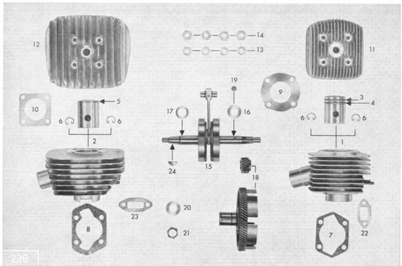
Tafel 5/1 Zylinder, Kurbeltrieb
