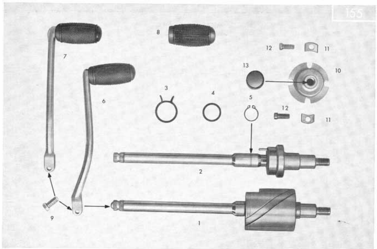
Tafel 21/1 Fußschaltwelle, Fußschalthebel
