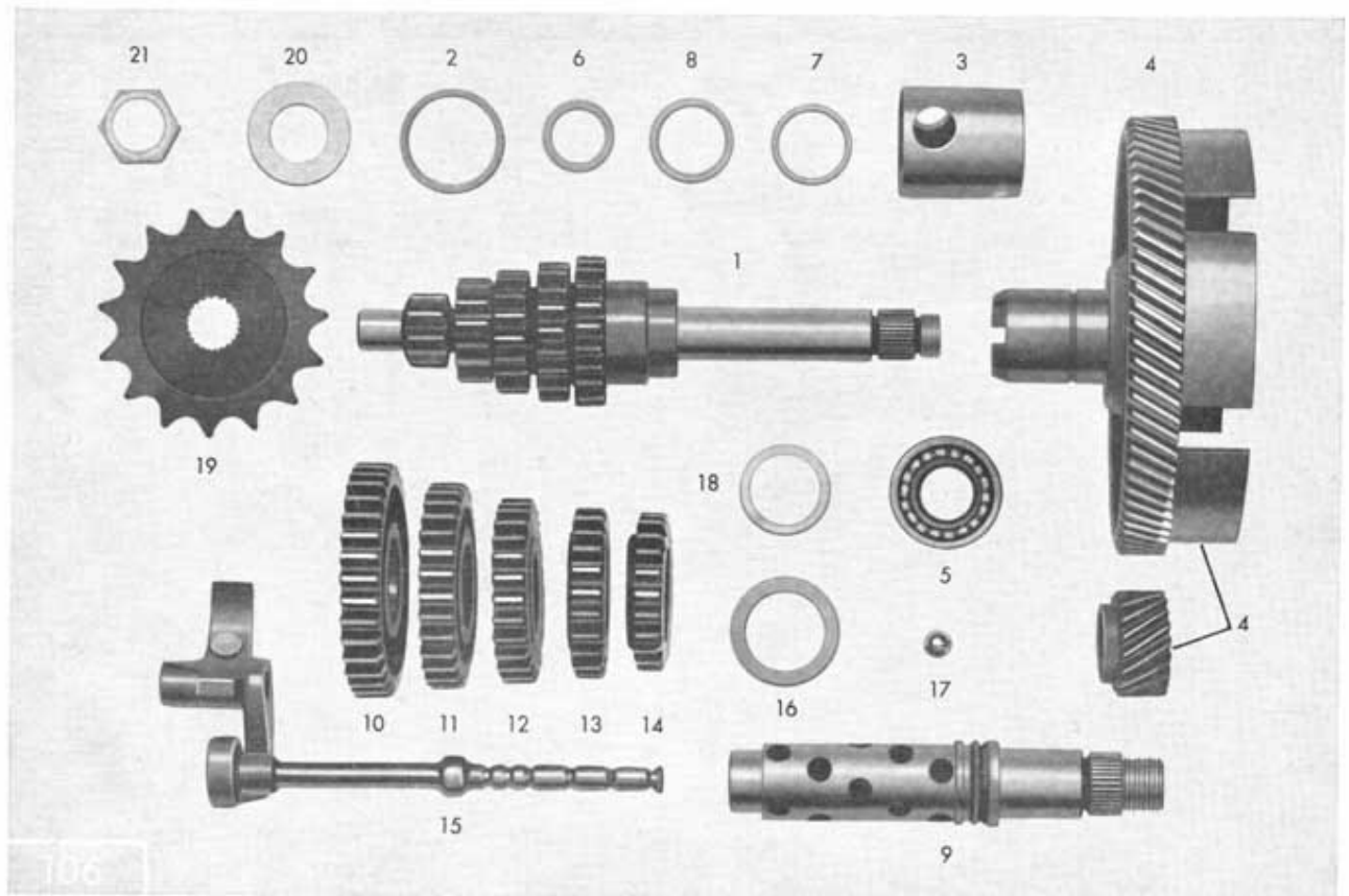
Tafel 19/1 Getriebewelle, Schaltwelle, Ziehkeil, Kettenritzel
