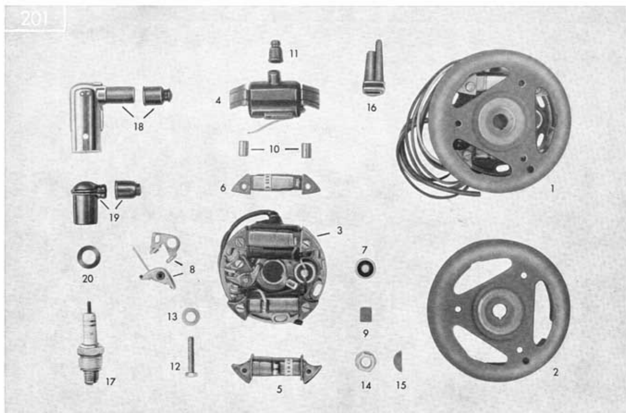
Tafel 11/1 Elektrische Ausrüstung
