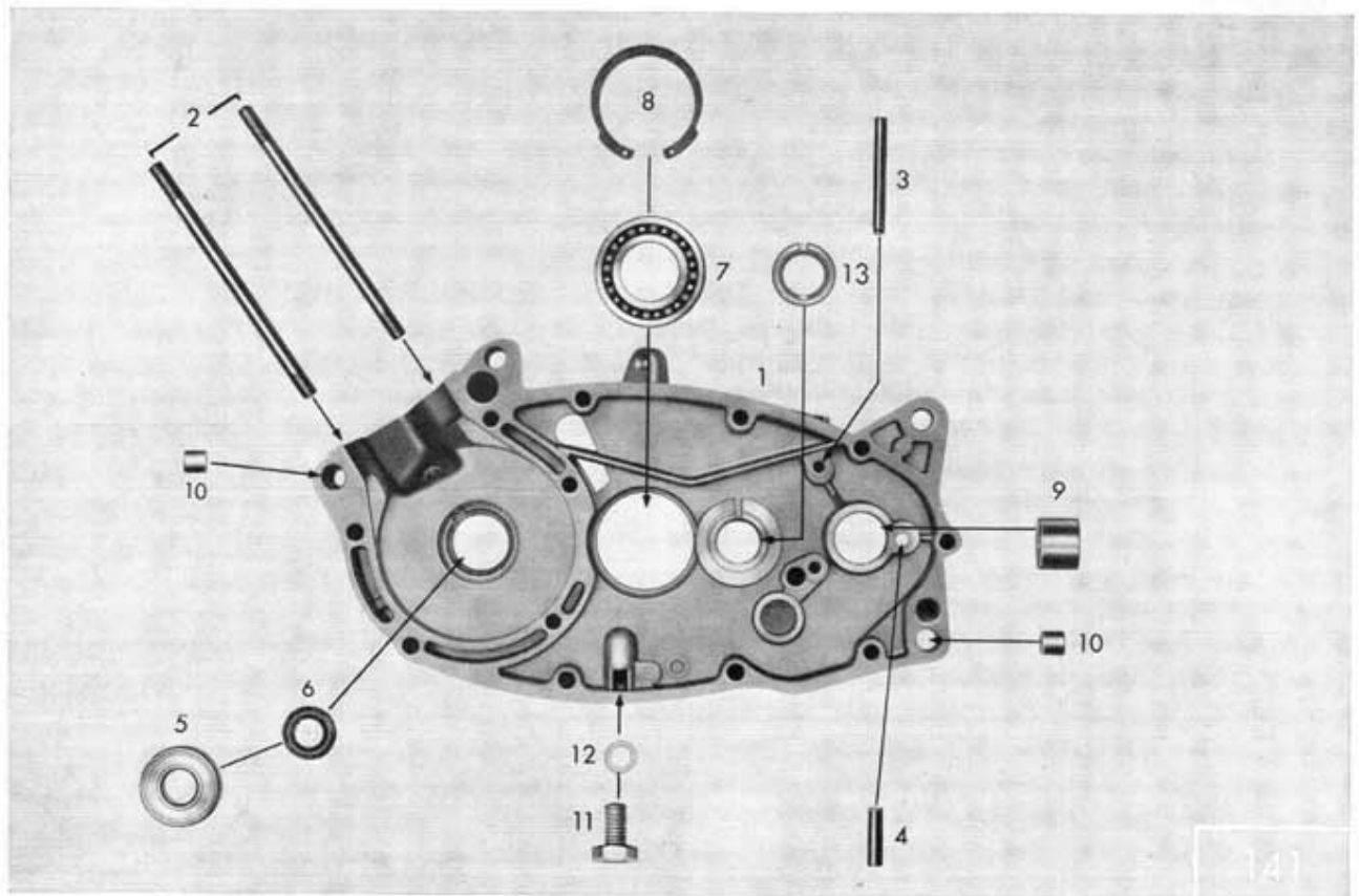
Tafel 1/1 Gehäusehälfte rechts
