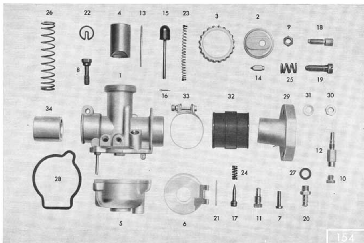
Tafel 18/3 Vergaser, Ansaugung
