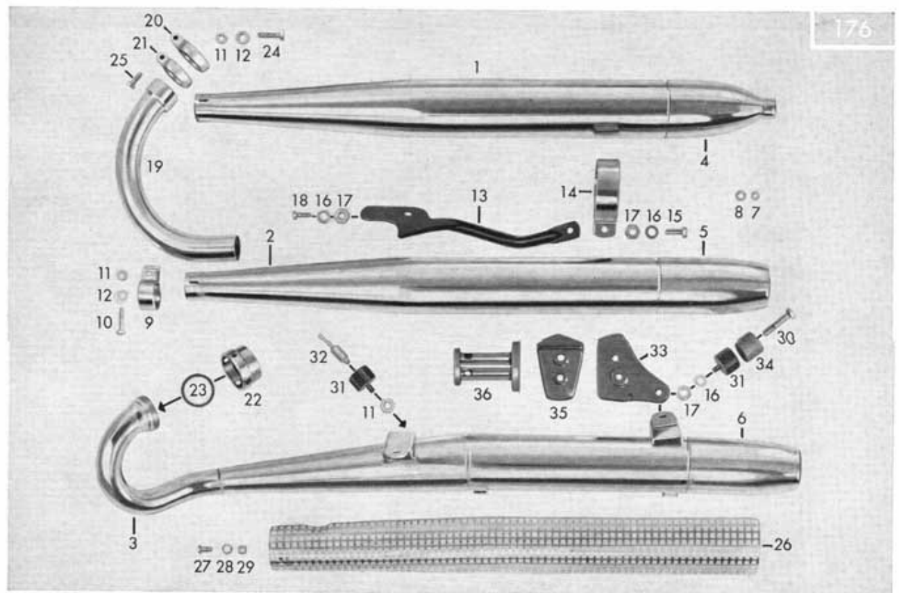
Tafel 24/2 Auspuff-Anlage
