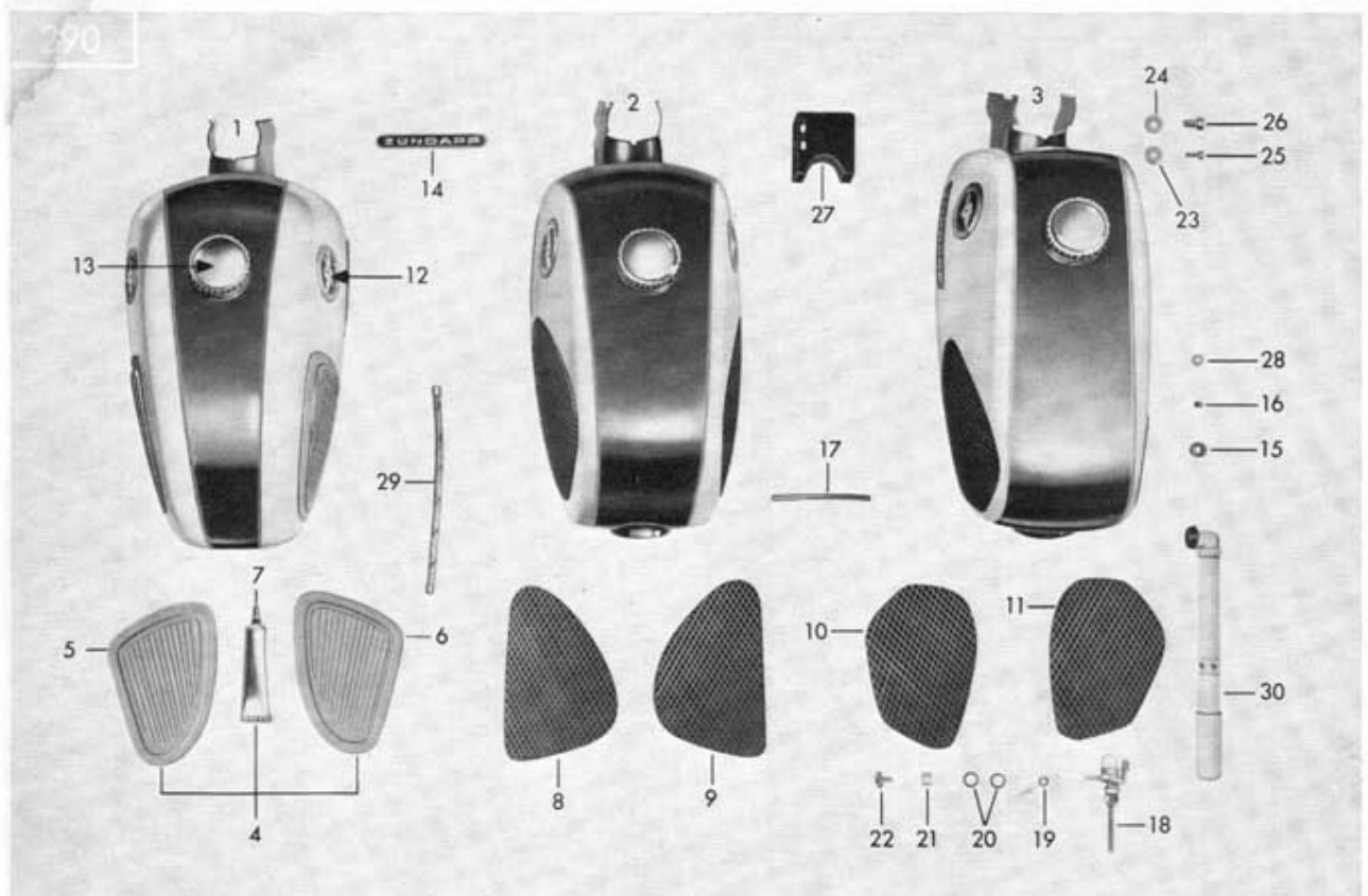
Tafel 37/1 Kraftstoffbehälter, Werkzeug-Satz
