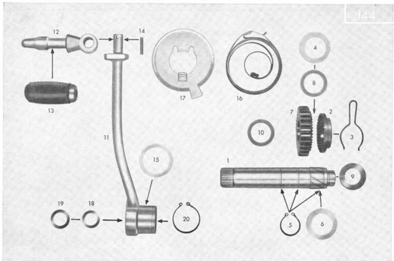
Tafel 8/1 Kickstarterwelle, Kickstarterhebel
