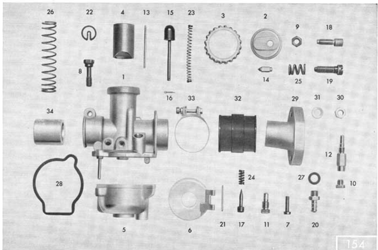
Tafel 18/2 Vergaser, Ansaugung
