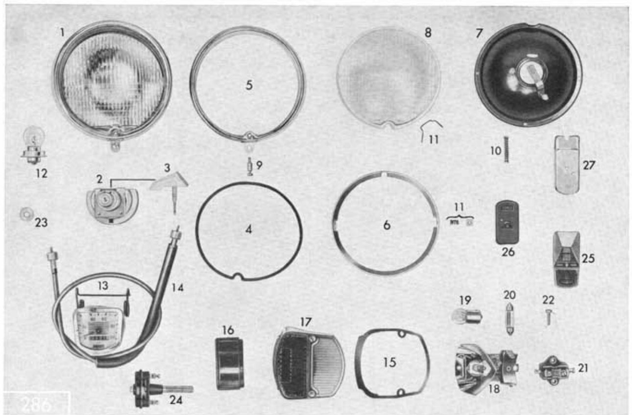
Tafel 34/2 Lichtanlage (dauerabgeblendet), Tachometer, Stopplicht
