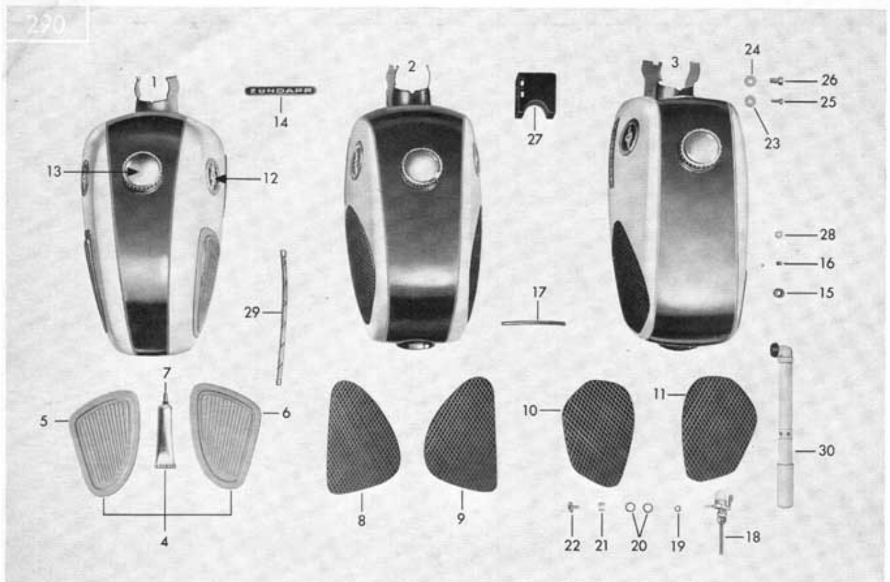
Tafel 37/2 Kraftstoffbehälter, Werkzeug-Satz
