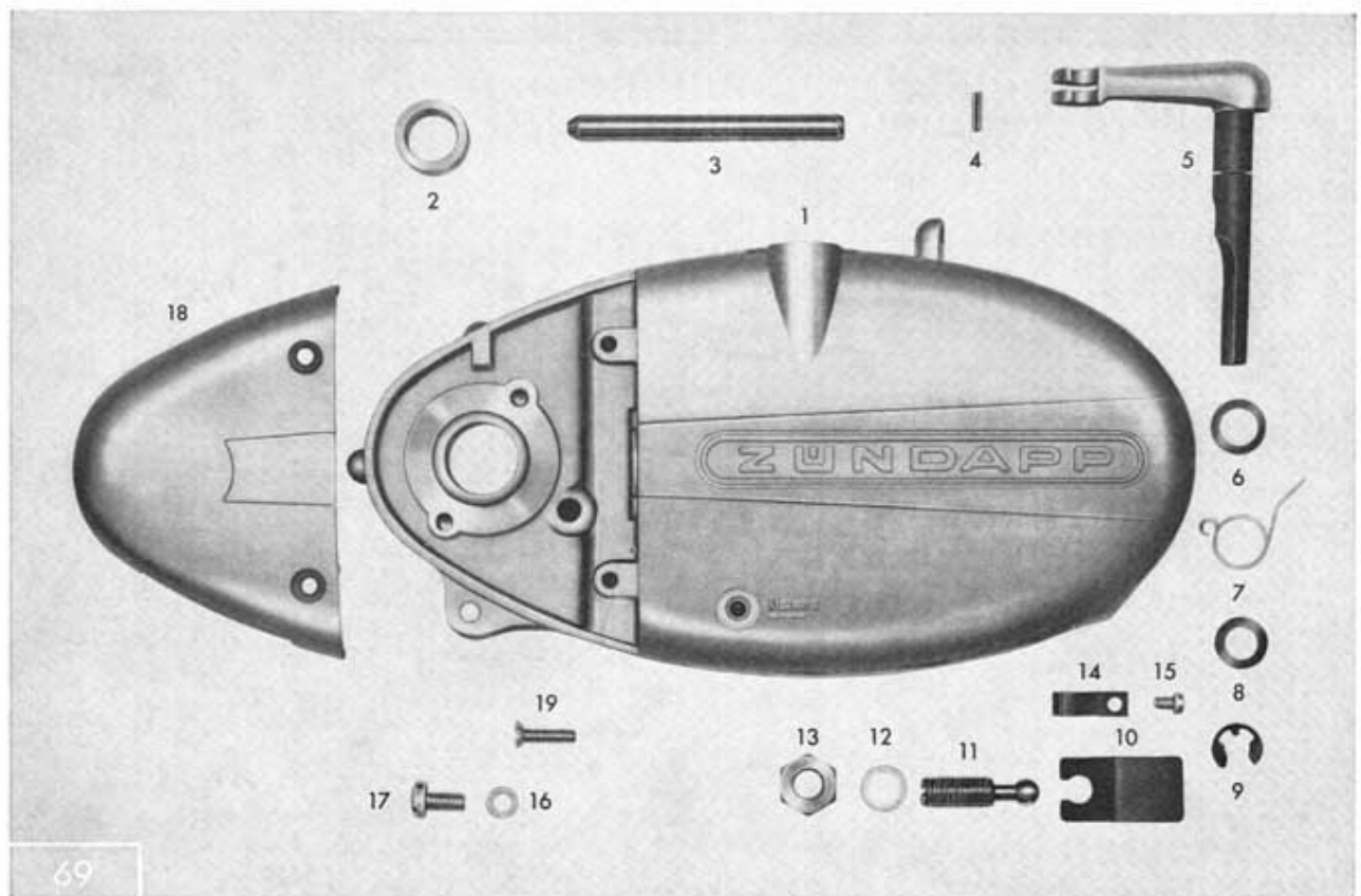
Tafel 16/1 Gehäusedeckel rechts, Kupplungshebel
