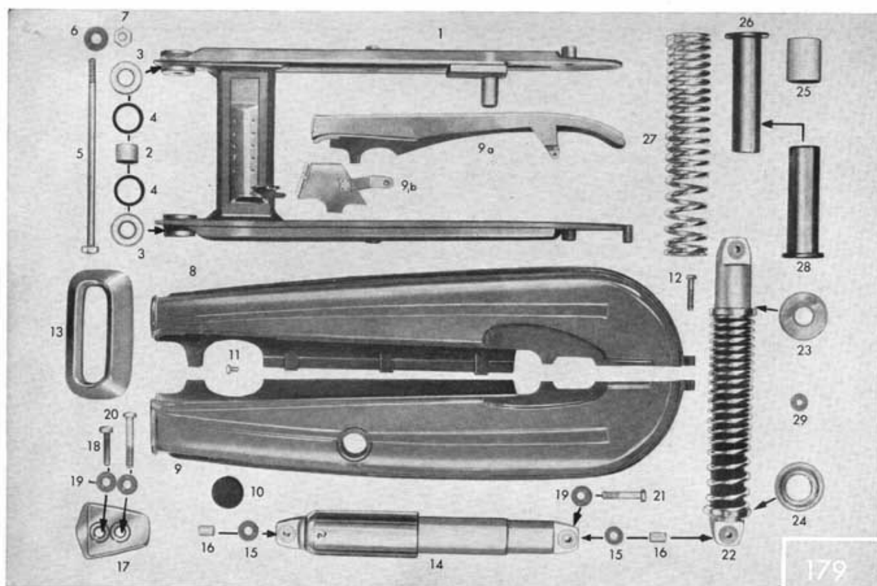
Tafel 28/2 Hinterradgabel, Federbein, Kettenschutz
