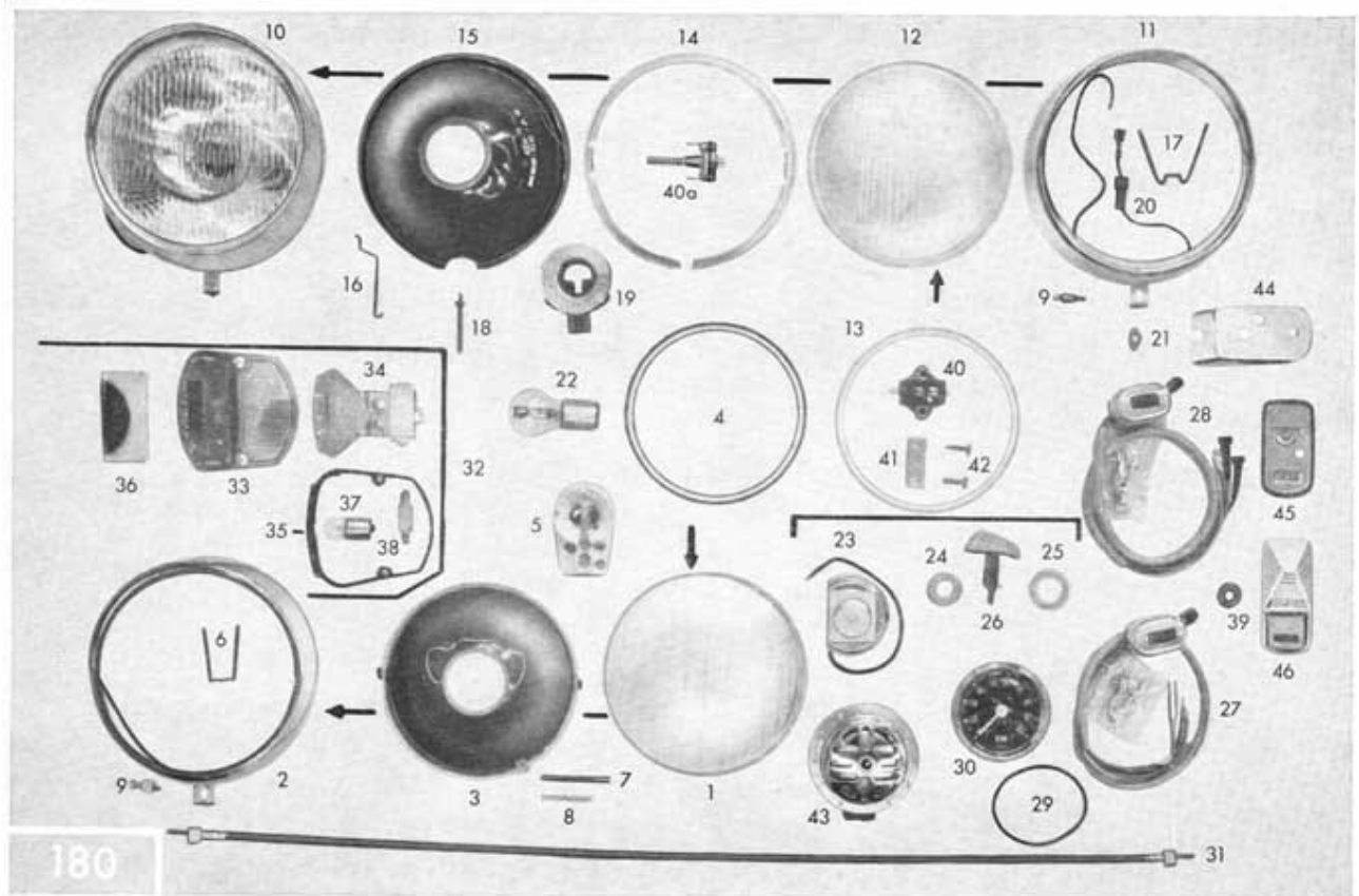
Tafel 33/3 Lichtanlage (25 W Bilux), Tachometer, Stopplight
