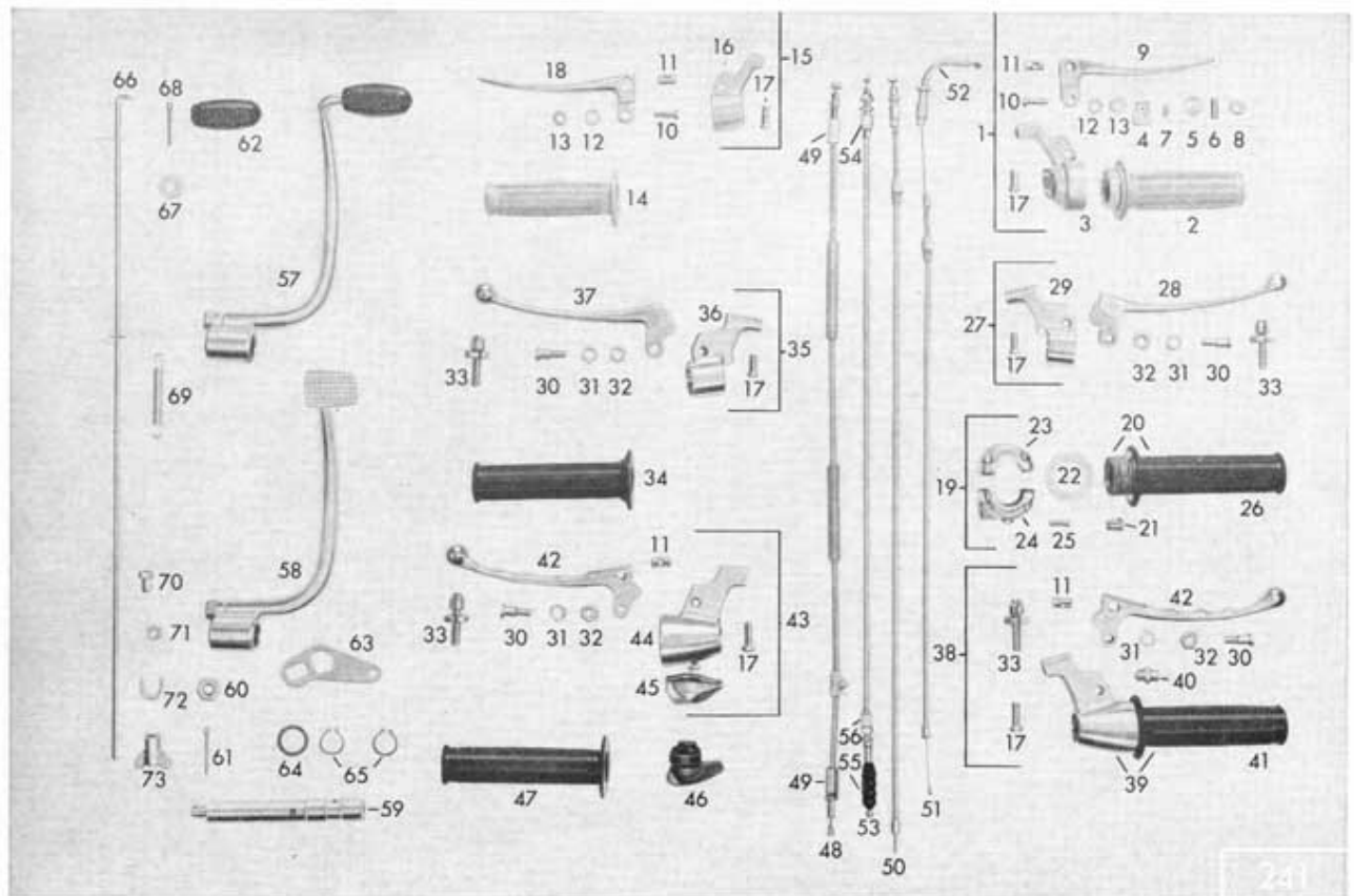
Tafel 35/2 Sport-Armaturen, bis Fahrgestell-Nr. 5 599 478
