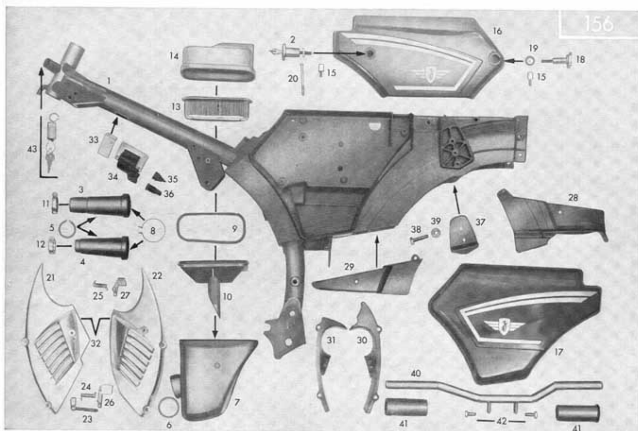
Tafel 25/1 Rahmen, Ansauggeräuschdämpfer, Vergaserverkleidung, Fußrastenrohr
