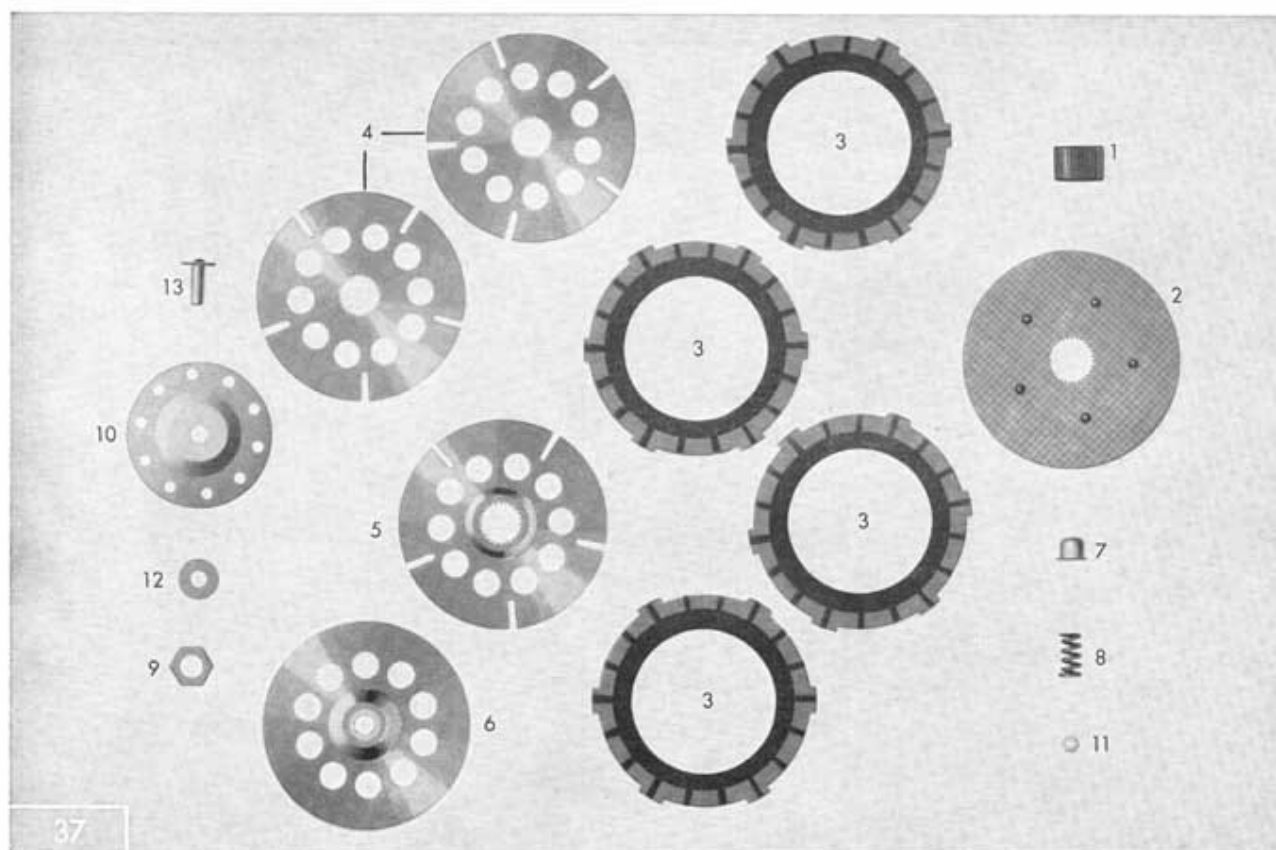
Tafel 10/1 Kupplung
