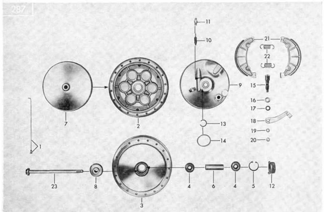
Tafel 30/2 Vorderes Laufrad, Vorderradnabe 150 mm \phi
