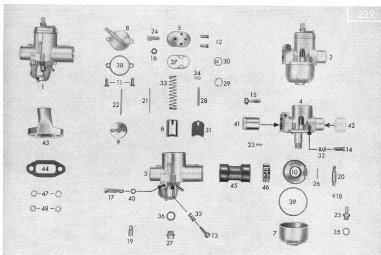
Tafel 6/2 Vergaser, Ansaugung
