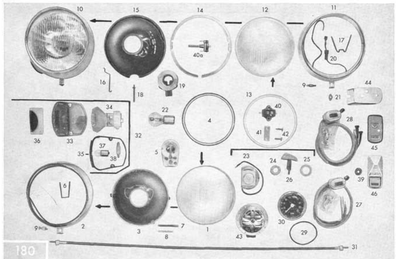
Tafel 33/2 Lichtanlage (25 W Bilux), Tachometer, Stopplicht
