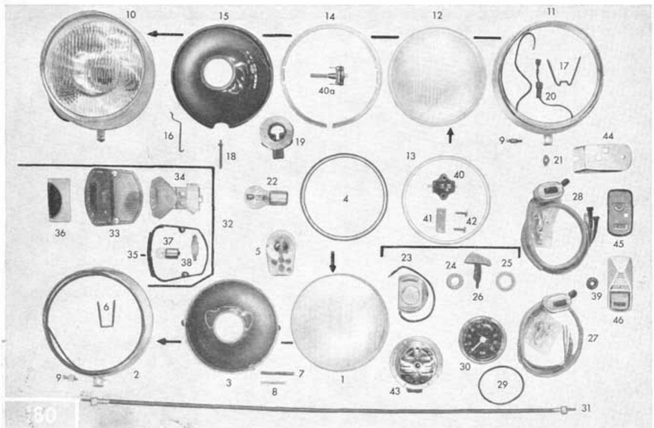
Tafel 33/1 Lichtanlage (25 W Bilux), Tachometer, Stopplicht
