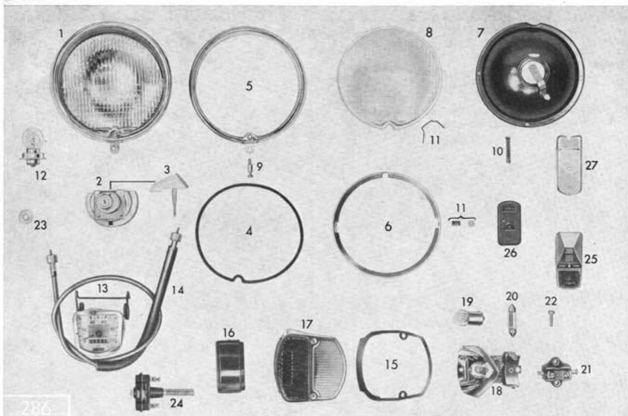
Tafel 34/1 Lichtanlage (dauerabgeblendet), Tachometer, Stopplicht
