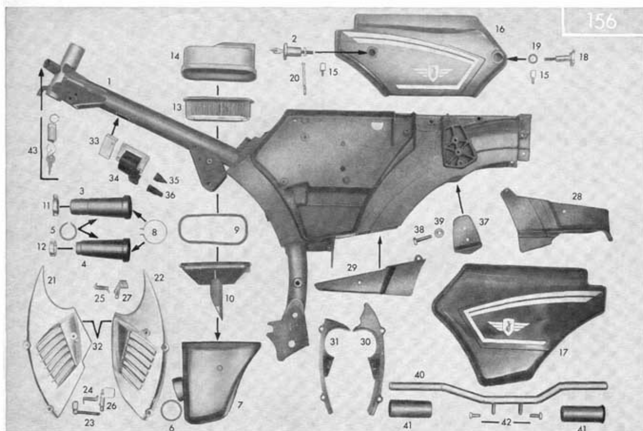
Tafel 25/2 Rahmen, Ansauggeräuschkämpfer, Vergaserverkleidung, Fußrastenrohr
