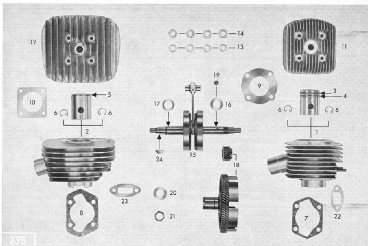
Tafel 5/2 Zylinder, Kurbeltrieb
