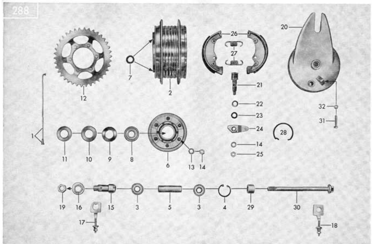
Tafel 31/1 Hinteres Laufrad, Hinterradnabe 120 mm \phi
