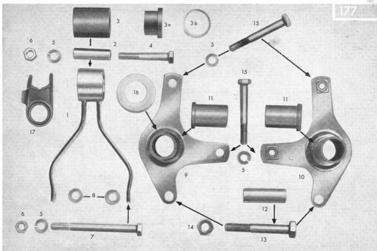
Tafel 26/1 Motoraufhängung, Motorträger
