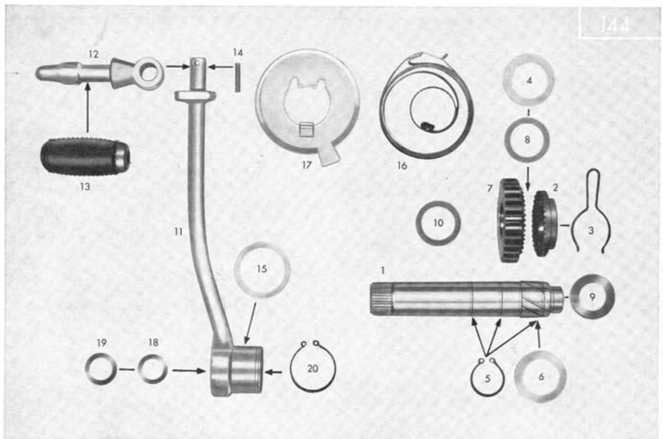
Tafel 20/1 Kickstarterwelle, Kickstarterhebel
