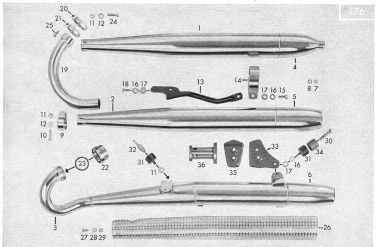
Tafel 24/1 Auspuff-Anlage
