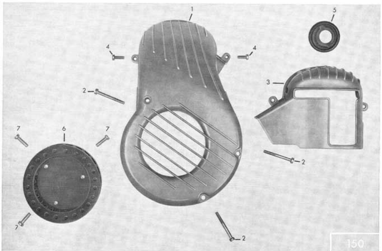
Tafel 15/1 Lüftergehäuse, Lüfterrad
