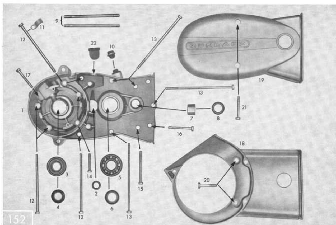
Tafel 14/1 Gehäusehälfte links, Gehäusedeckel links
