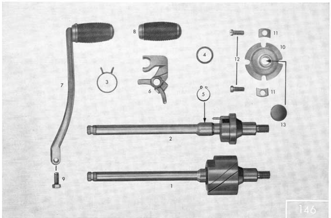
Tafel 9/1 Fußschaltwelle, Fußschalthebel
