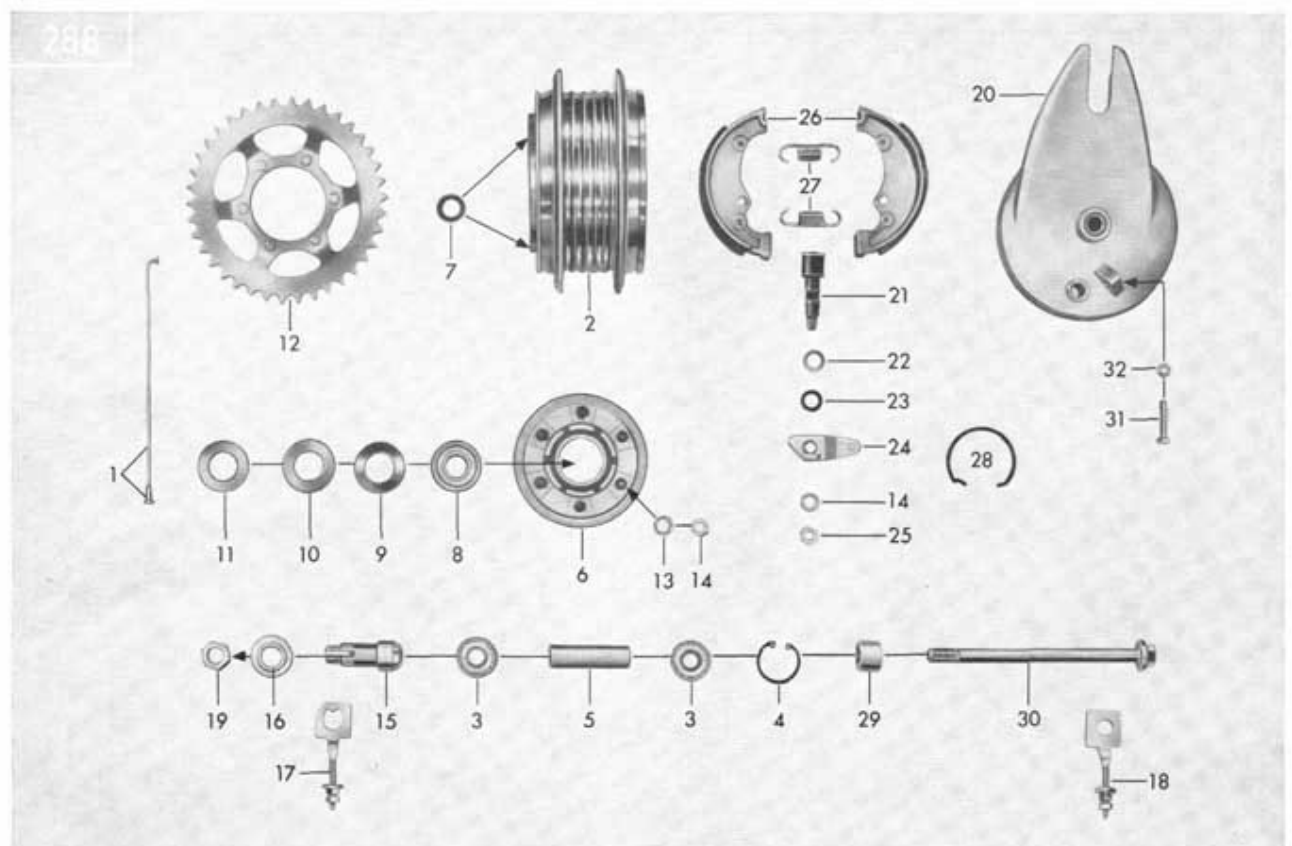
Tafel 31/2 Hinteres Laufrad, Hinterradnabe 120 mm \phi
