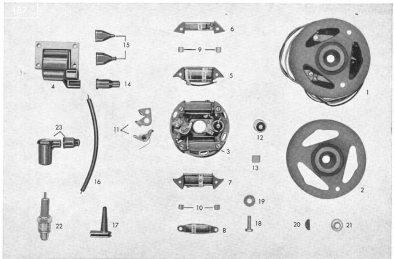
Tafel 23/1 Elektrische Ausrüstung (Zündspule außenliegend)
