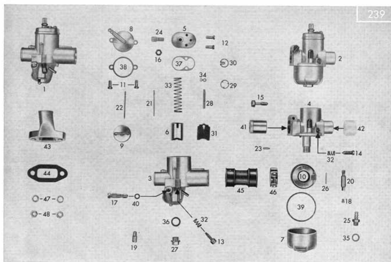
Tafel 6/1 Vergaser, Ansaugung
