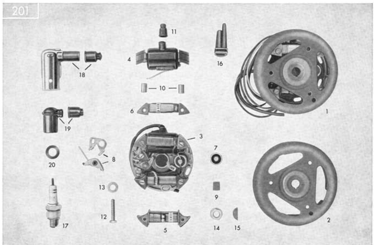
Tafel 23/2 Elektrische Ausrüstung (Zündspule innenliegend)
