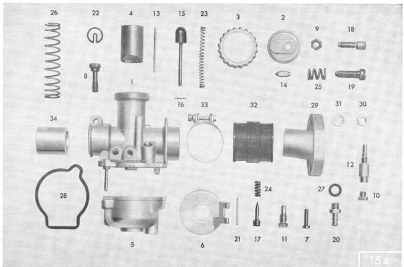
Tafel 18/1 Vergaser, Ansaugung
