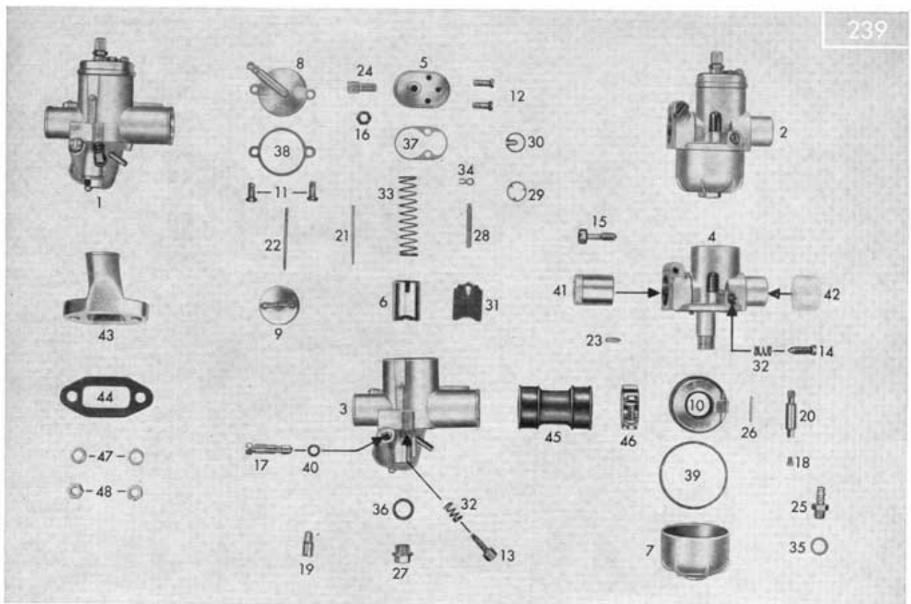
Tafel 6/3 Vergaser, Ansaugung
