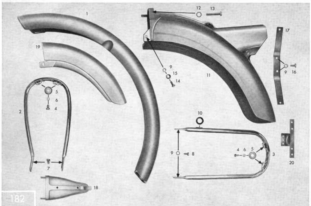
Tafel 36/1 Schutzbleche, Zierbügel, Nummernschildhalter
