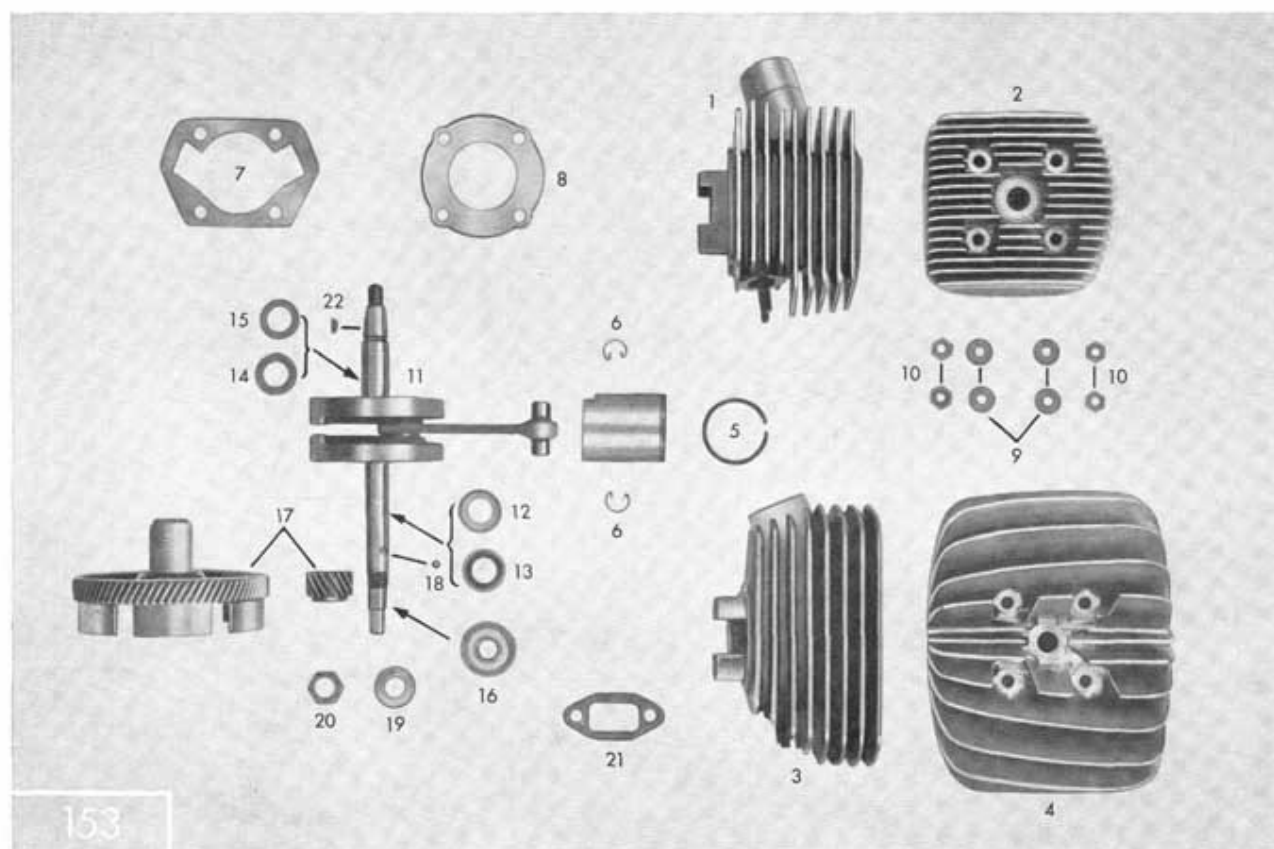
Tafel 17/2 Zylinder, Kurbeltrieb
