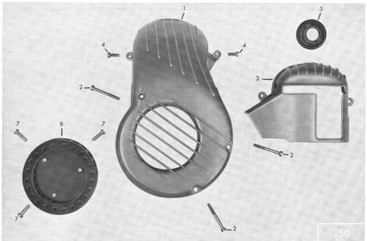
Tafel 3/1 Lüftergehäuse, Lüfterrad
