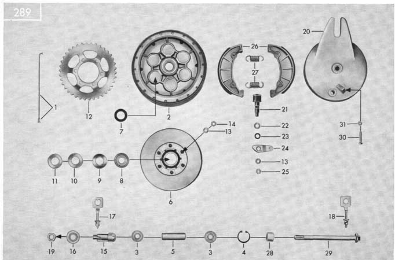
Tafel 32/2 Hinteres Laufrad, Hinterradnabe 150 mm \phi
