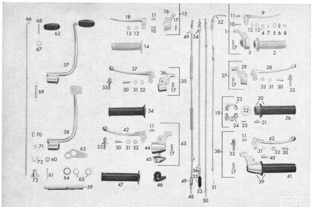
Tafel 35/3 Sport-Armaturen, ab Fahrgestell-Nr. 5 599 479
