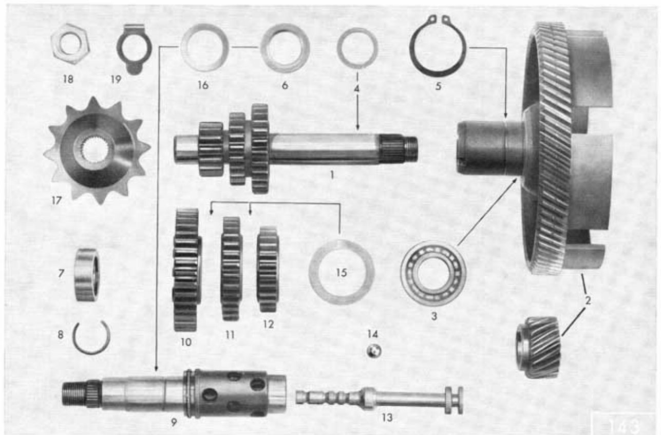
Tafel 7/1 Getriebewelle, Schaltwelle, Ziehkeil, Kettenritzel
