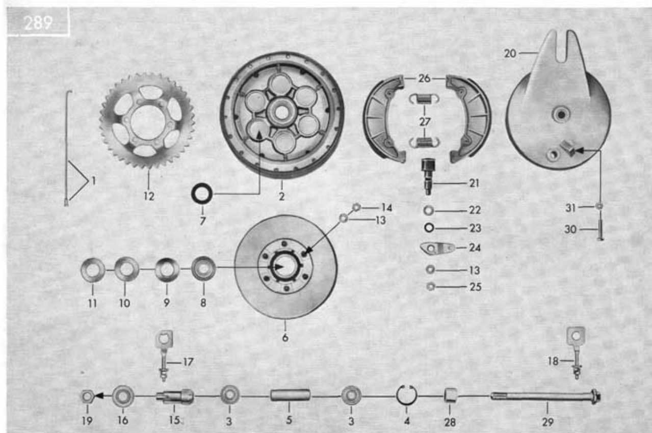
Tafel 32/1 Hinteres Laufrad, Hinterradnabe 150 mm \phi
