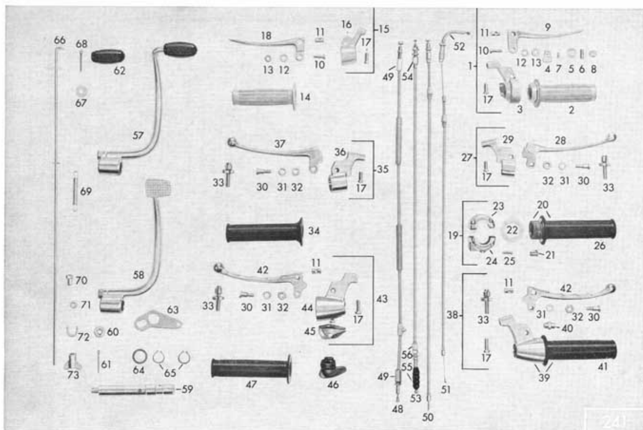
Tafel 35/1 Normal-Armaturen
