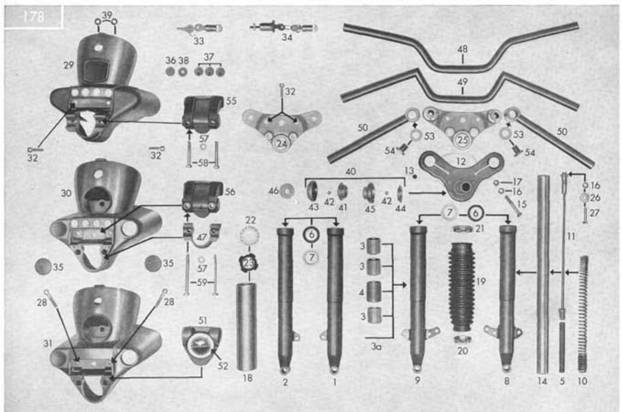
Tafel 27/1 Vorderradgabel, Gabelgehäuse, Lenkungslager, Lenker
