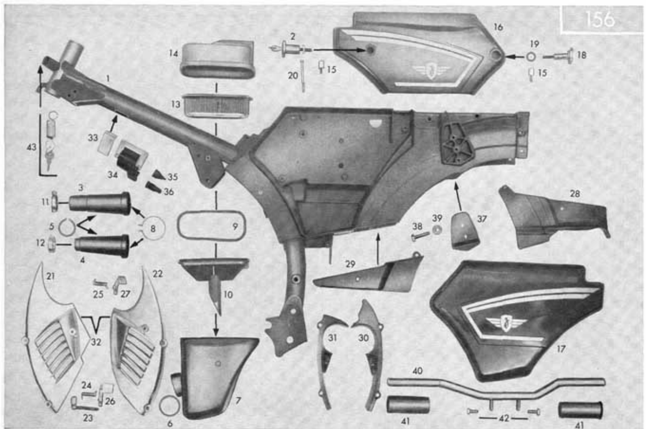
Tafel 25/3 Rahmen, Ansauggeräuschdämpfer, Vergaserverkleidung, Fußrastenrohr
