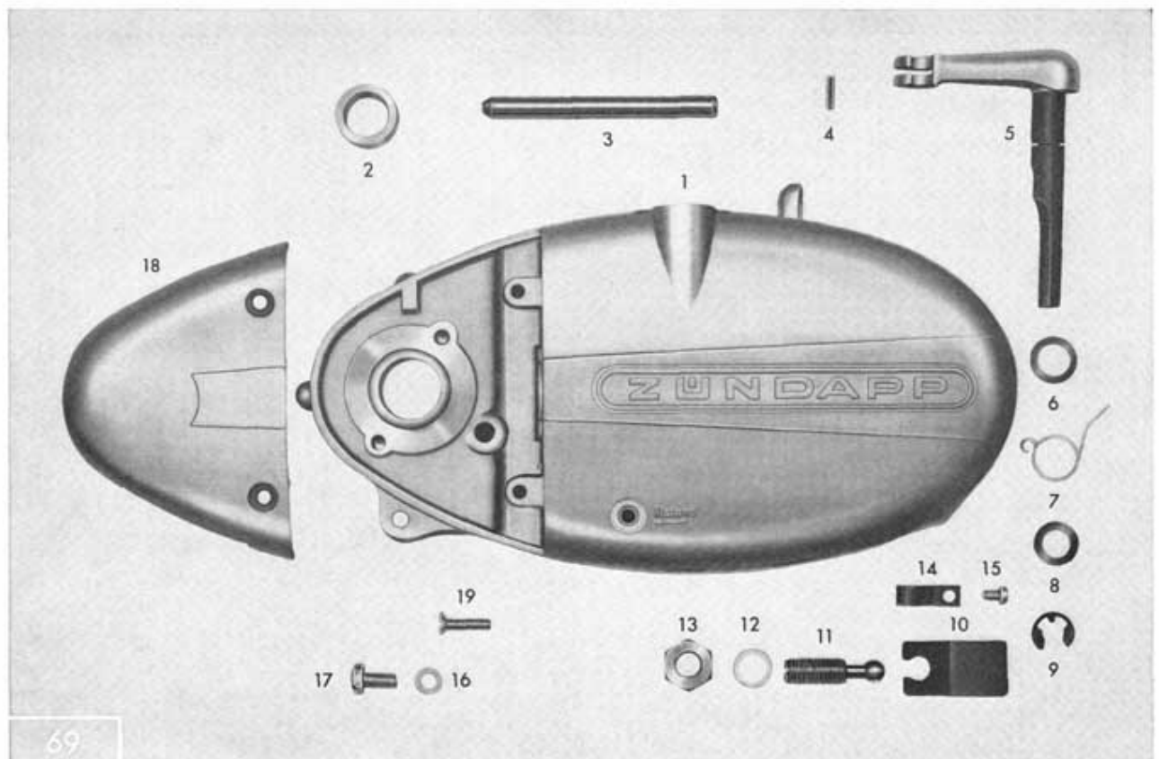
Tafel 4/1 Gehäusedeckel rechts, Kupplungshebel
