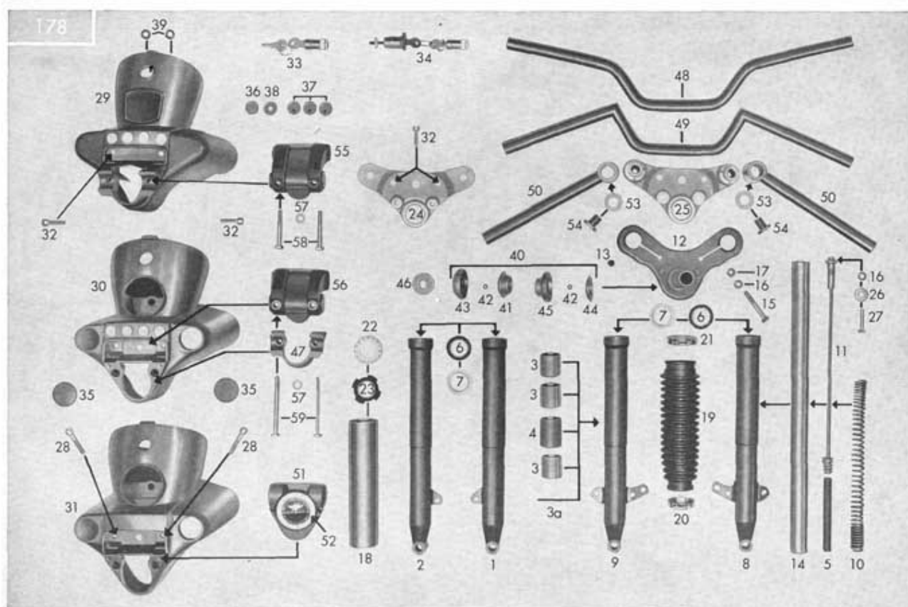
Tafel 27/2 Vorderradgabel, Gabelgehäuse, Lenkungslager, Lenker
