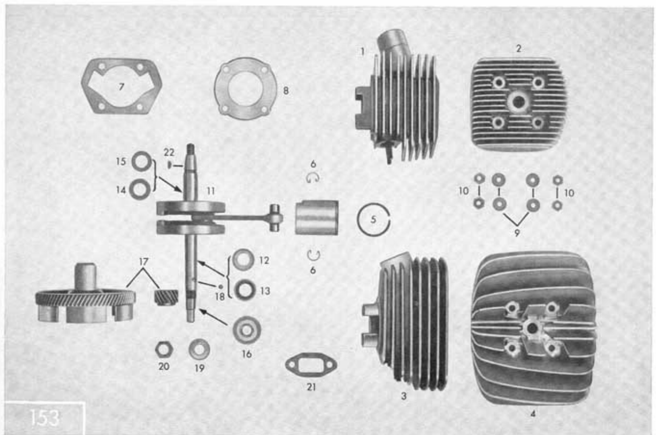
Tafel 17/1 Zylinder, Kurbeltrieb
