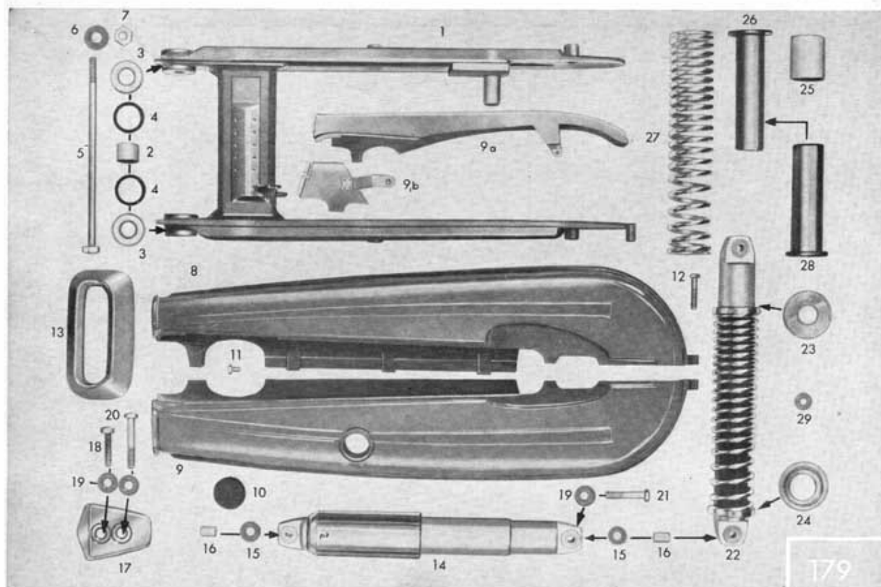
Tafel 28/1 Hinterradgabel, Federbein, Kettenschutz
