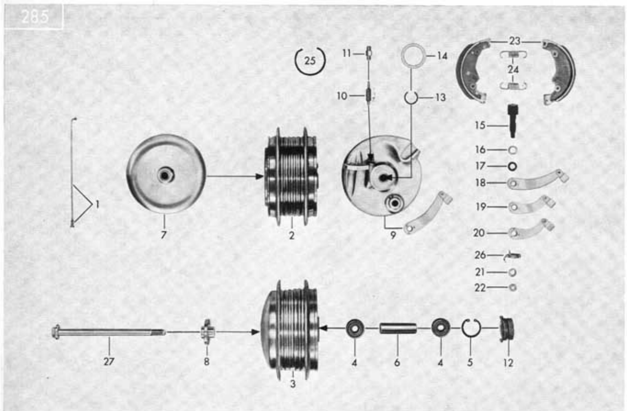
Tafel 29/1 Vorderes Laufrad, Vorderradnabe 120 mm \phi
