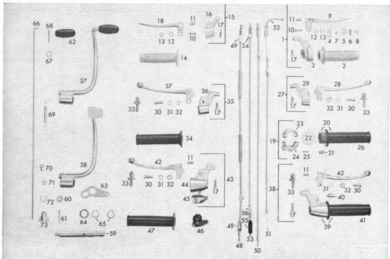
Tafel 35/4 Seilzüge für Normal- und Sport-Armaturen
