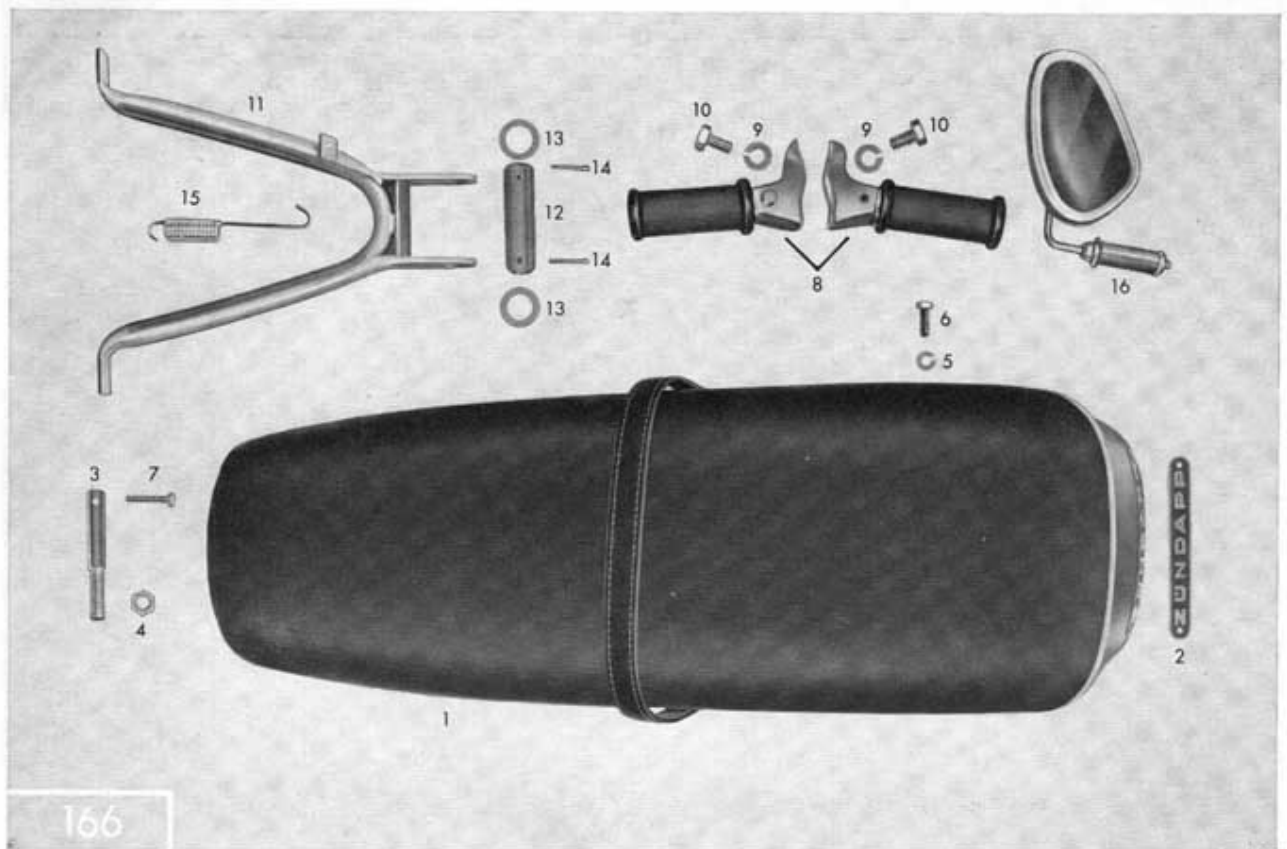
Tafel 38/1 Doppelsitzbank, Radständer, Fußrasten, Spiegel
