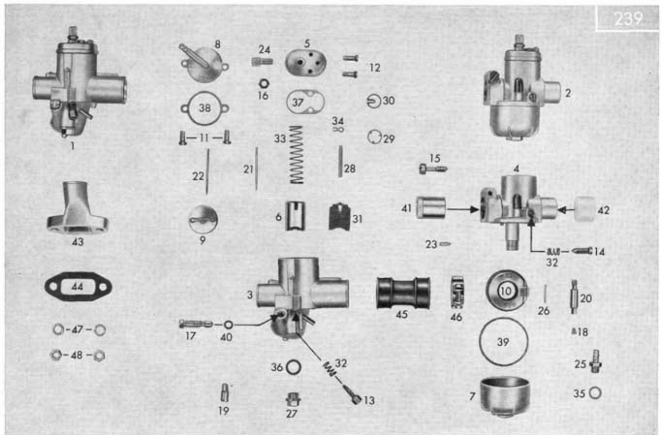
Tafel 6/4 Vergaser, Ansaugung
