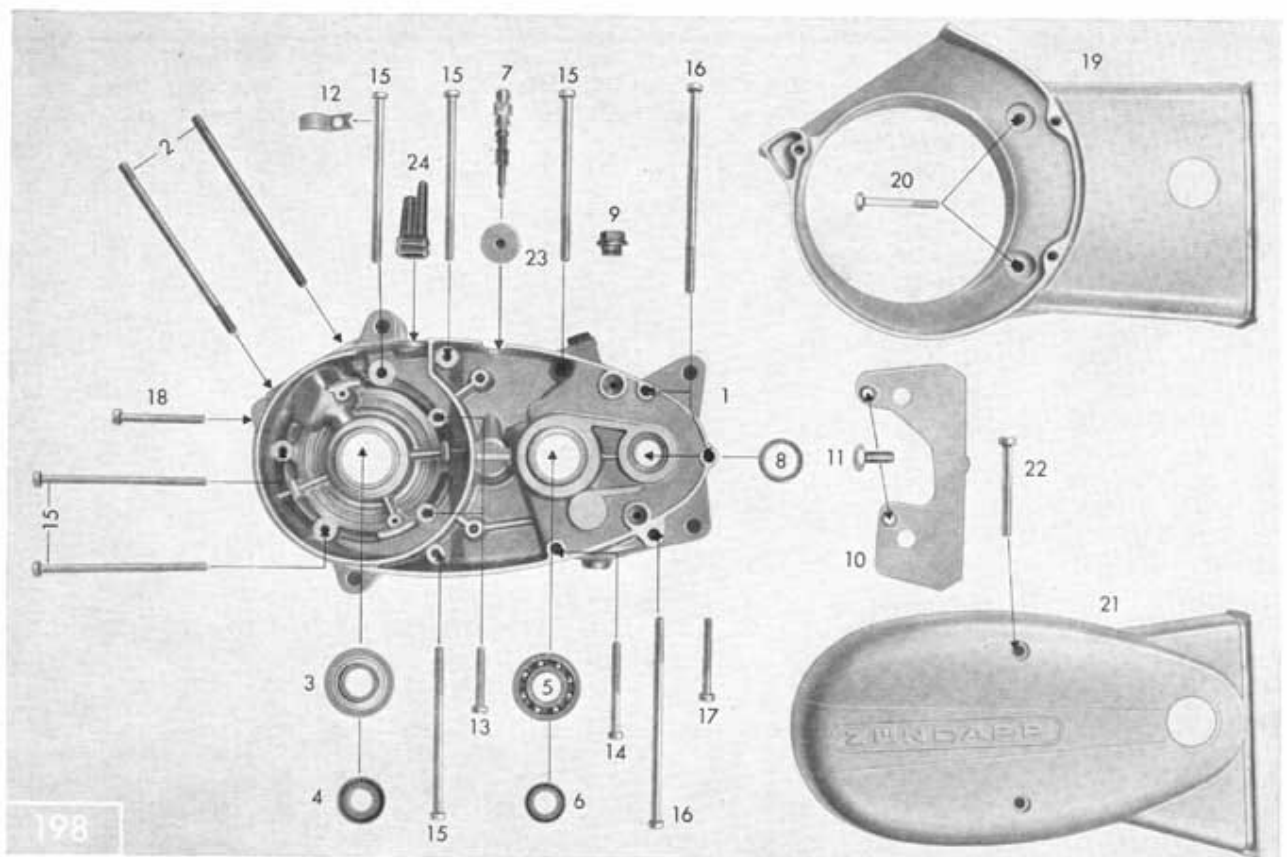
Tafel 2/1 Gehäusehälfte links, Gehäusedeckel links
