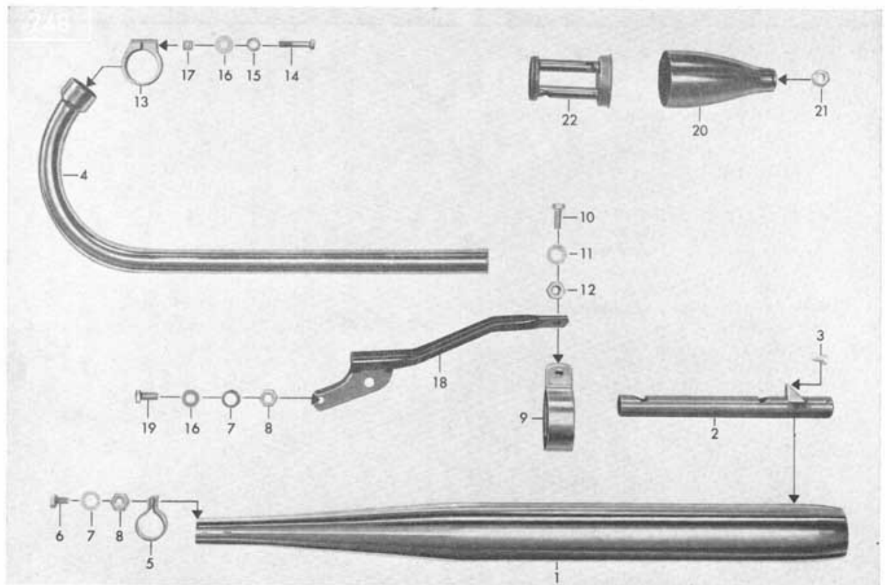
Tafel 12/1 Auspuff-Anlage
