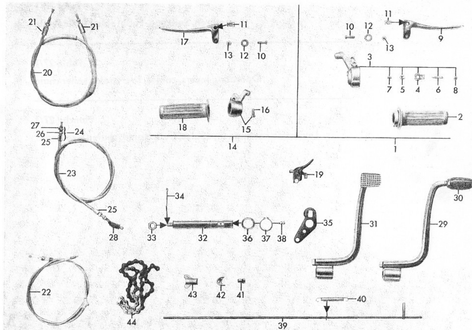
Tafel 27/1 Armaturen, Seilzüge, Fußbremse, Rollenkette Table 27/1 Operating levers, cables, foot brake, roller chain Planche 27/1 Leviers de commande, câbles, frein à pied, chaîne à rouleaux
