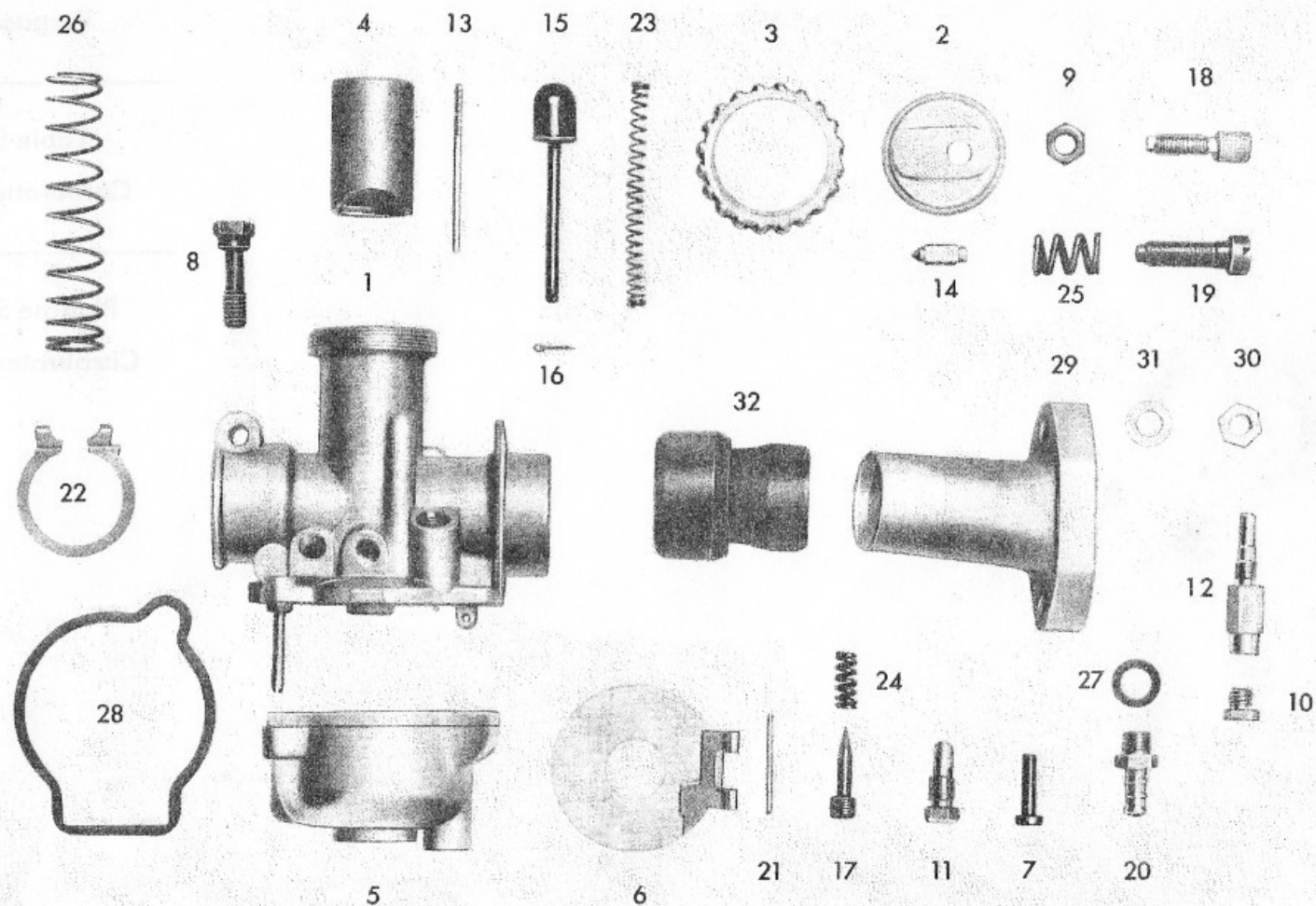
Tafel 5a Vergaser Table 5a Carbu­rettor Planche 5a Carburateur
