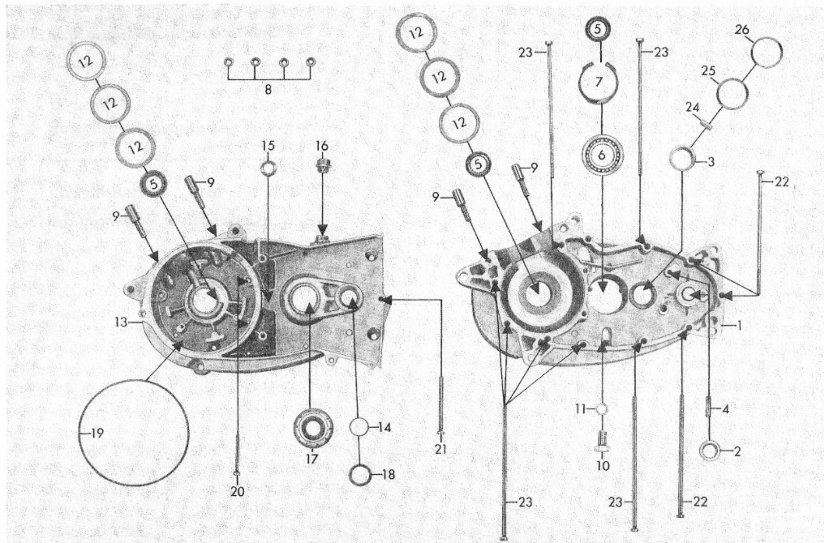
Planche 12/1 Carter droite, carter gauche
