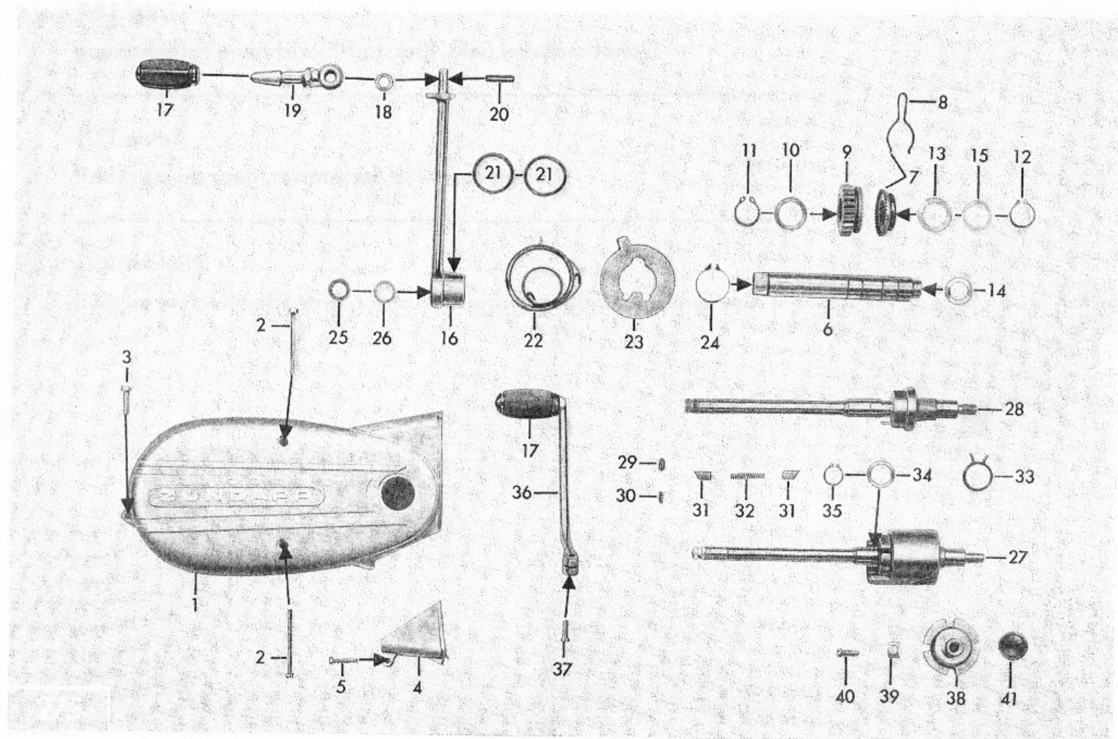
Tafel 13/1 Gehäusedeckel links, Kickstart-Einrichtung, Fußschaltung Table 13/1 Casing cover left, kickstarter, gear change shaft Planche 13/1 Couvercle de carter gauche, kickstarter, arbre de sélecteur au pied
