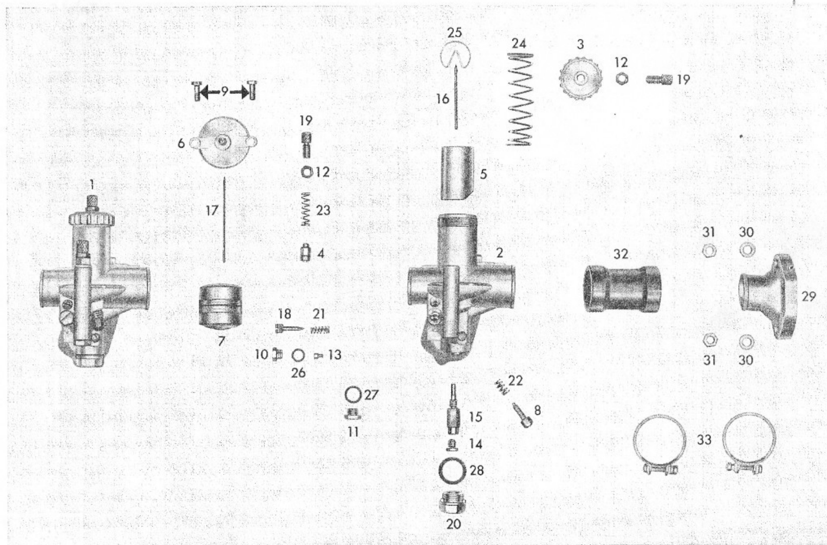
Tafel 5 Vergaser Table 5 Carburettor Planche 5 Carburateur
