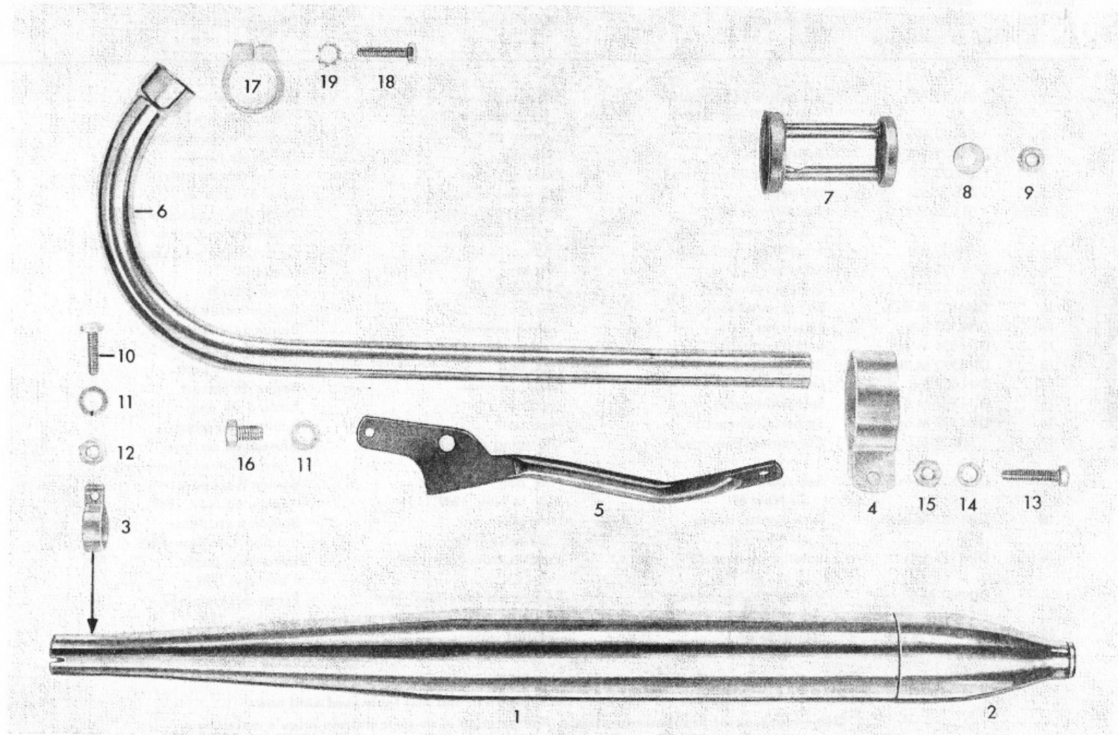
Tafel 11 Auspuff Table 11 Exhaust Planche 11 Système d'échappement
