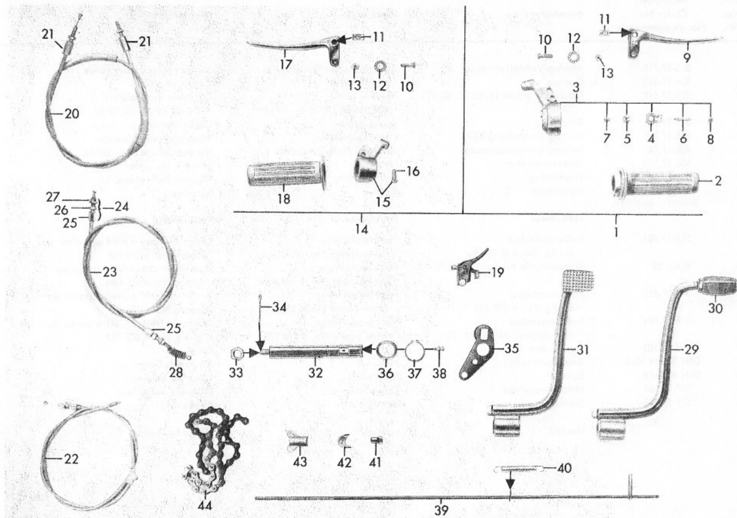
Tafel 27/2 Armaturen, Seilzüge, Fußbremse, Rollenkette Table 27/2 Operating levers, cables, foot brake, roller chain Planche 27/2 Leviers de commande, câbles, frein à pied, chaîne à rouleaux
