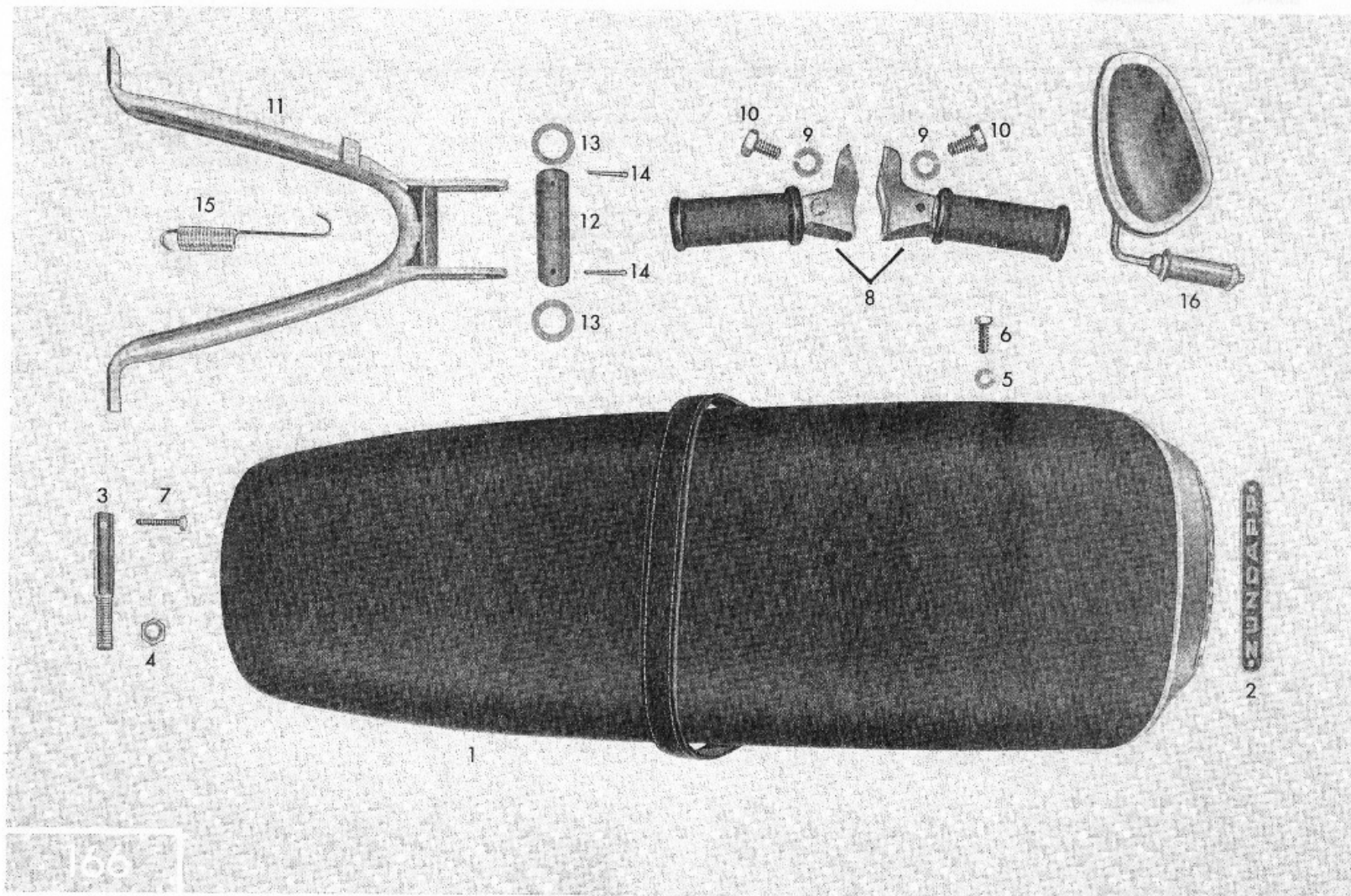
Tafel 30/1 Sitzbank, Radständer, Fußrasten, Spiegel Table 30/1 Bench seat, centre prop, foot-rests, rear view mirror Planche 30/1 Siège, béquille, repose-pieds, rétroviseur
