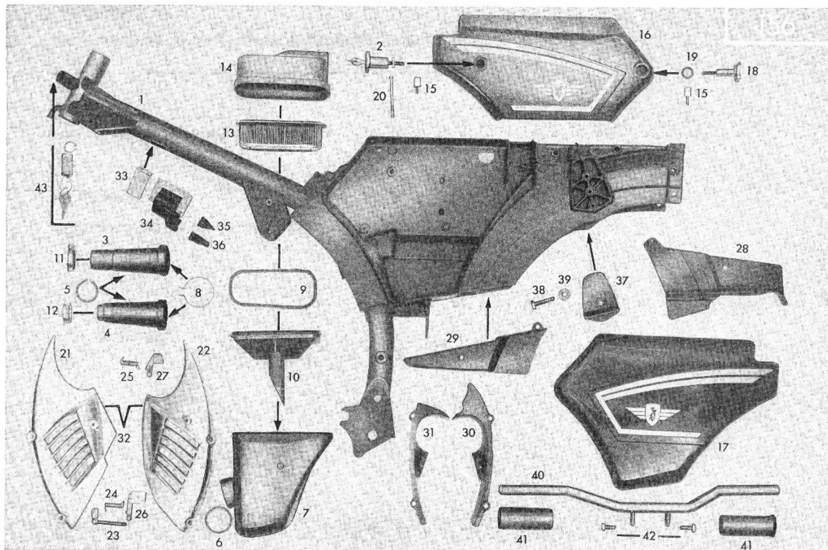
Tafel 19/1 Rahmen, Geräuschkämpfer, Deckel, Verkleidungen Table 19/1 Frame, noise damper, cover, fairings Planche 19/1 Cadre, amortisseur de bruit, couvercle, carénages
