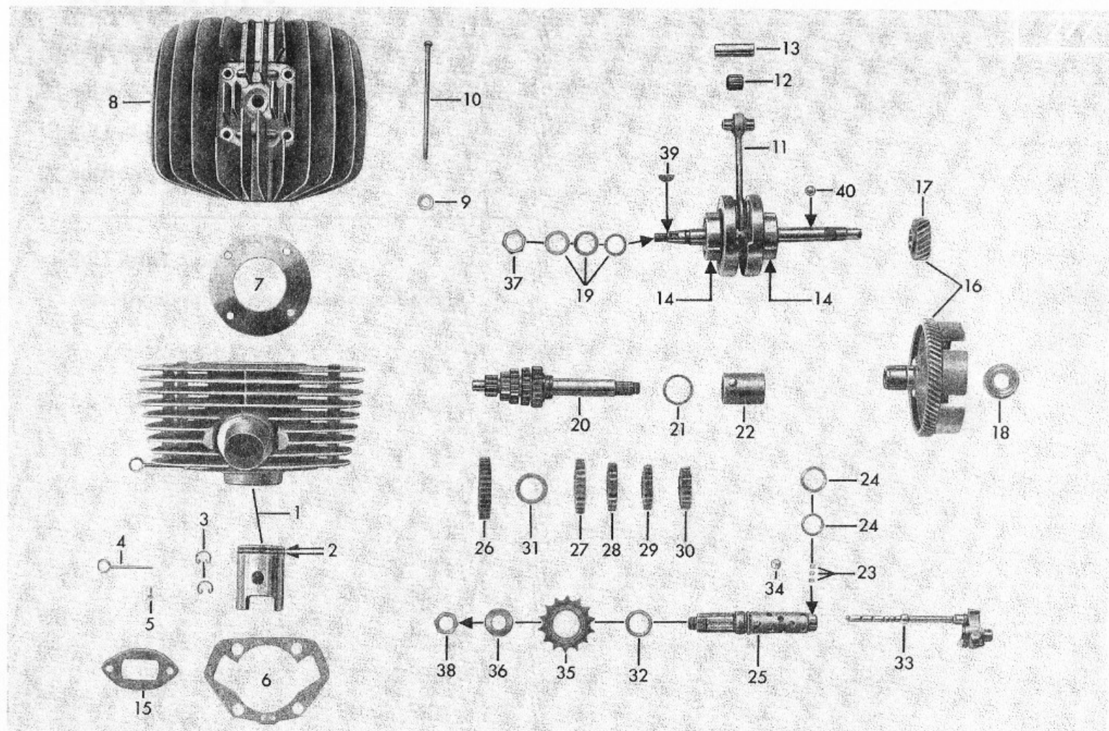
Tafel 15/3 Zylinder, Kurbelwelle, Getriebe Table 15/3 Cylinder, crankshaft, gearbox Planche 15/3 Cylindre, vilebrequin, boîte de vitesses
