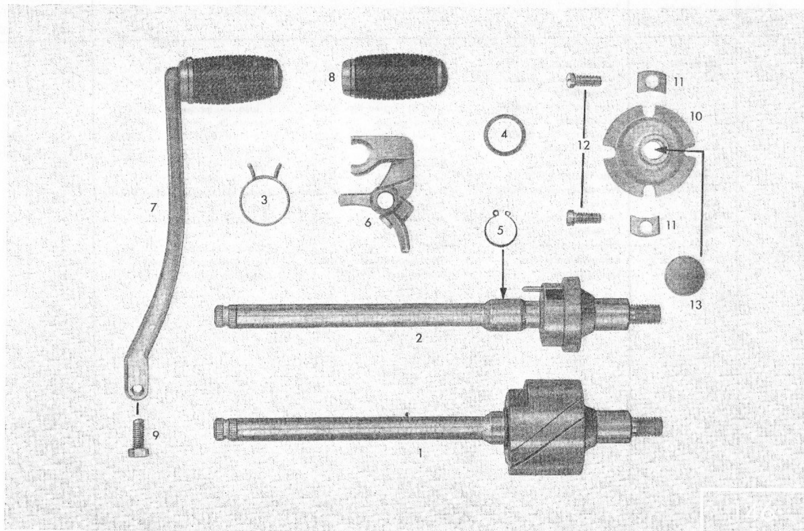
Tafel 8 Fußschaltwelle — Fußschalthebel Table 8 Gear Change Shaft — Pedal Planche 8 Arbre de sélecteur au pied — Levier de sélecteur au pied
