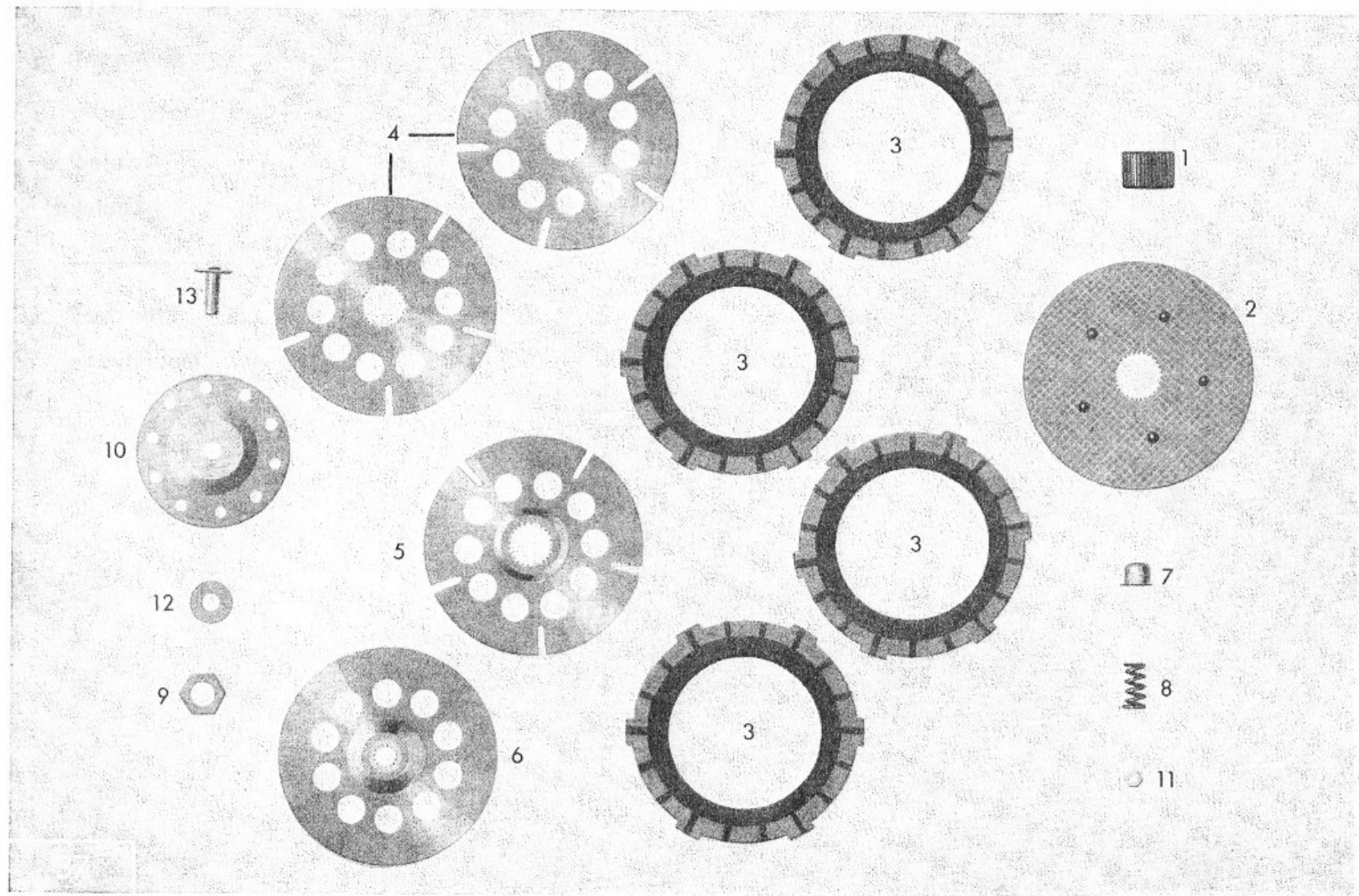
Tafel 9 Kupplung Table 9 Clutch Planche 9 Embrayage
