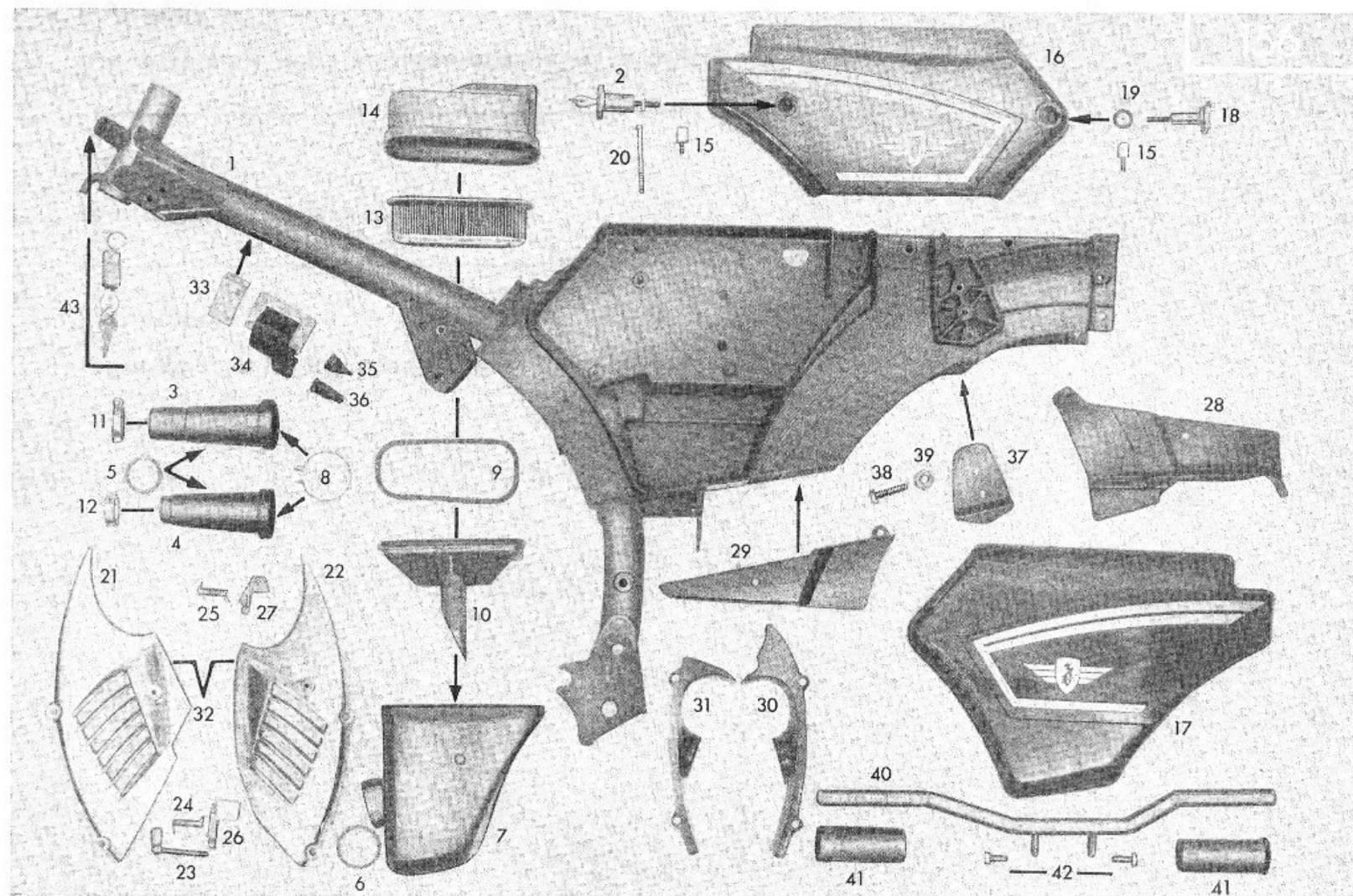
Tafel 19/2 Rahmen, Geräuschdämpfer, Deckel, Verkleidungen Table 19/2 Frame, noise damper, cover, fairings Planche 19/2 Cadre, amortisseur de bruit, couvercle, carénages
