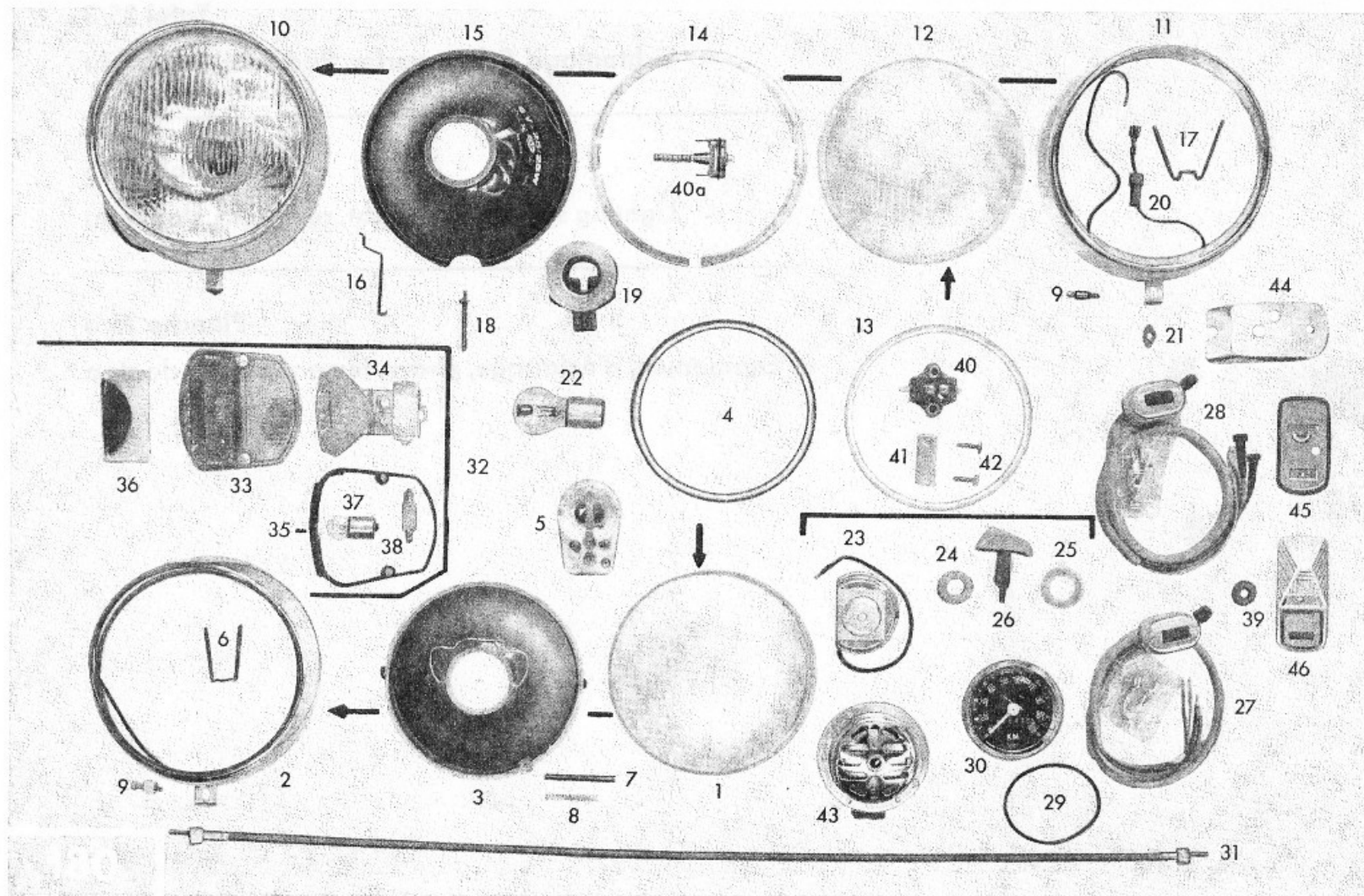
Tafel 25/3 Lichtanlage, Scheinwerfer, Rücklicht, Stopplight Table 25/3 Lighting System, headlight, rear Light, stop Light Planche 25/3 Equipement d'éclairage, phare, feu arrière, feu de stop
