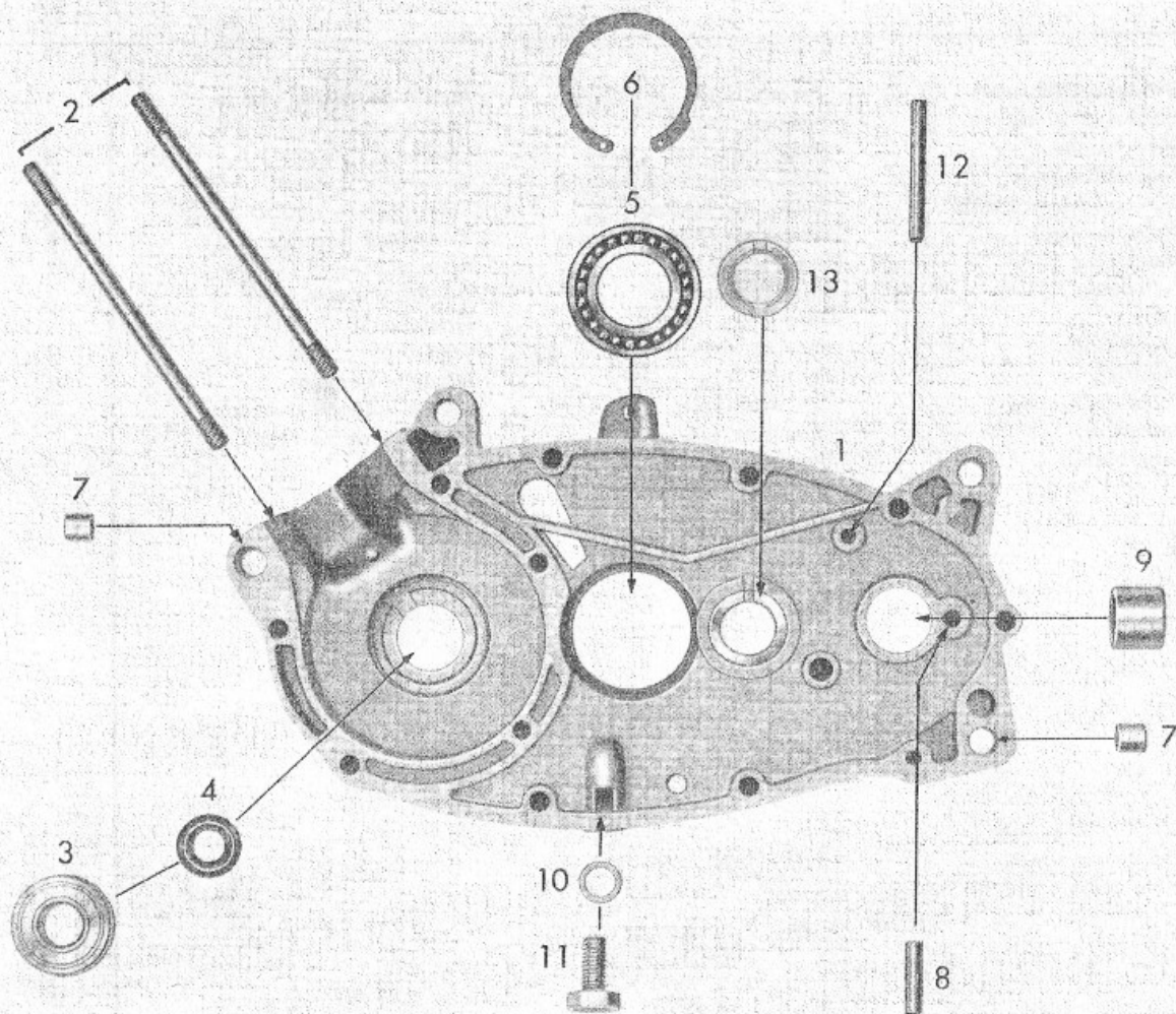
Tafel 1 Gehäusehälfte rechts Table 1 Casing, right Planche 1 Moitié de carter, droite
