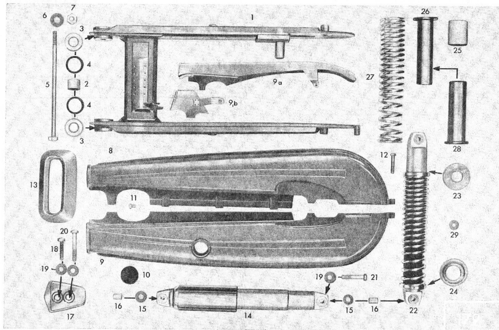
Tafel 22/1 Hinterradgabel, Kettenschutz, Federbein Table 22/1 Rear fork, chain guard, spring unit Planche 22/1 Fourche de roue AR, carter de chaîne, jambe à ressort
