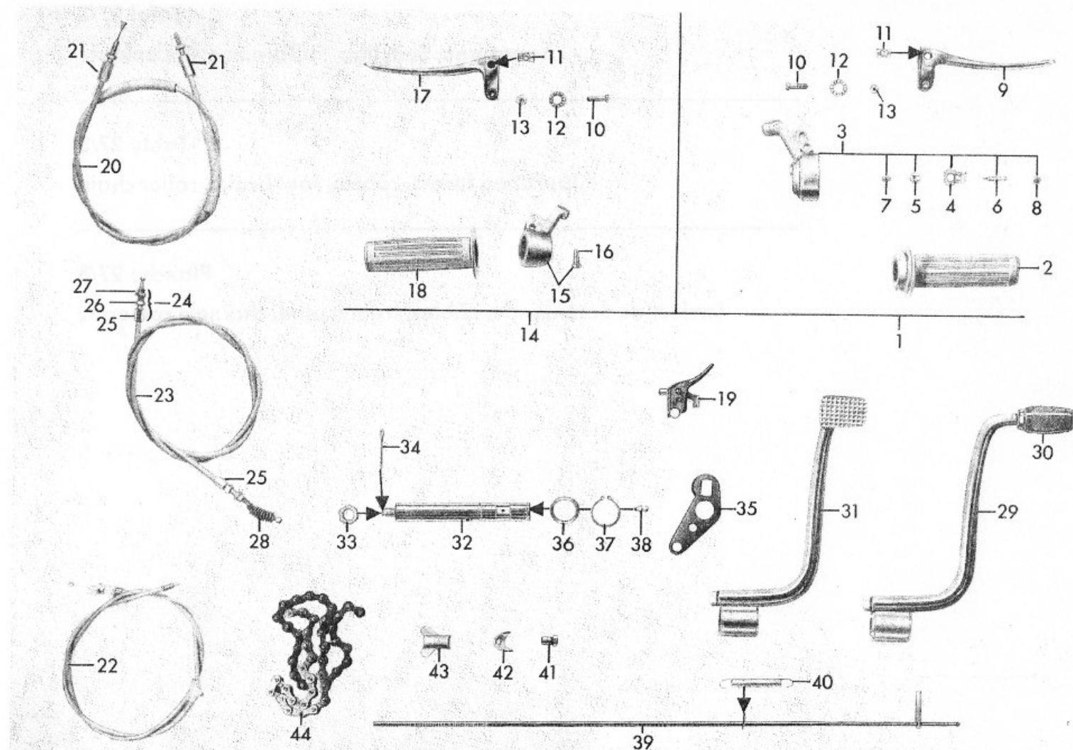
Tafel 27/3 Armaturen, Seilzüge, Fußbremse, Rollenkette Table 27/3 Operating levers, cables, foot brake, roller chain Planche 27/3 Leviers de commande, câbles, frein à pied, chaîne à rouleaux
