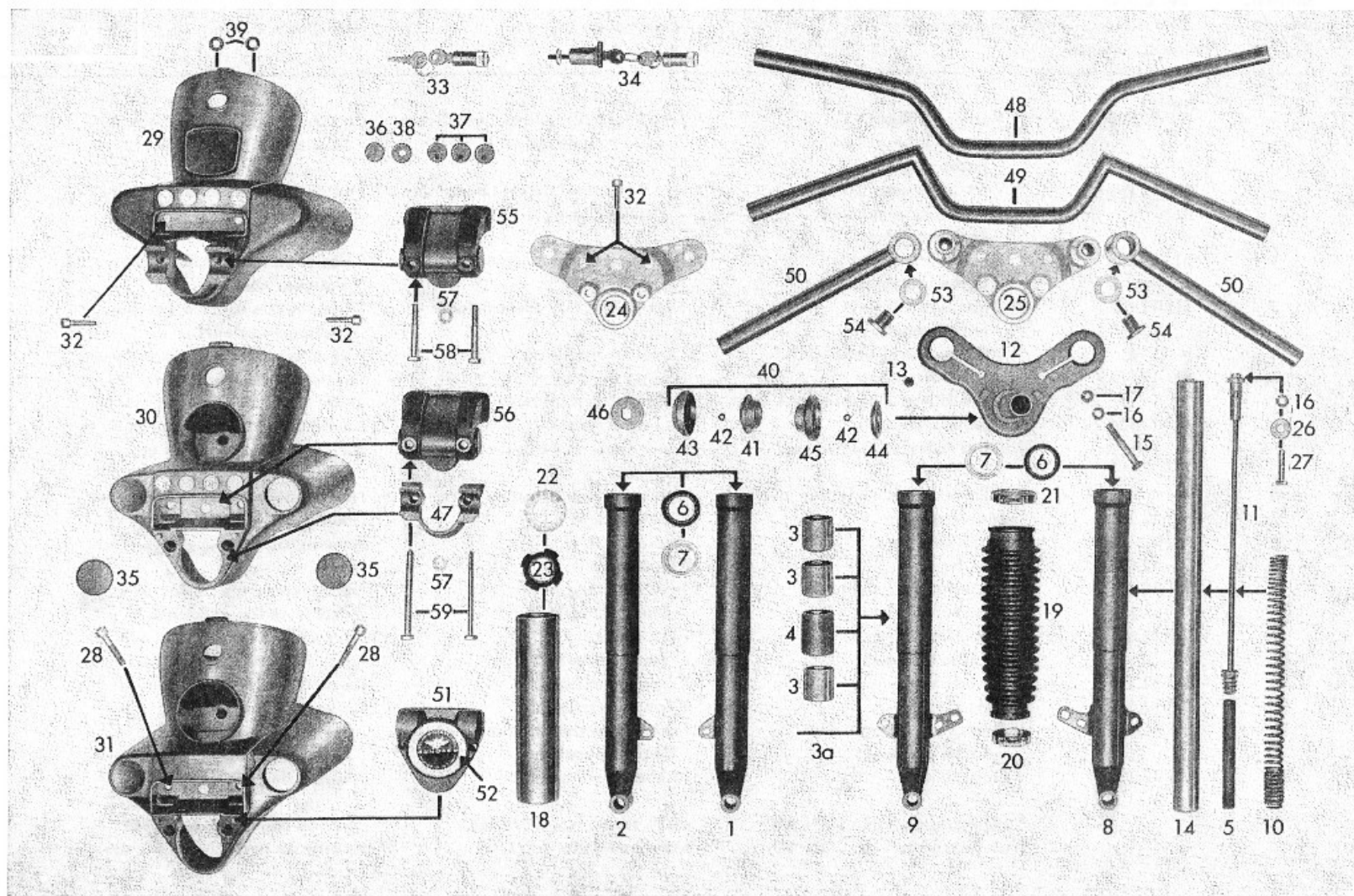
Tafel 21/1 Vorderradgabel – Gabelgehäuse – Lenkungslager – Lenker Table 21/1 Front fork – Headlamp casing – Handlebar bearing – Handlebar Planche 21/1 Fourche de roue AV – Coque de phare – Palier pour direction – Guidon
