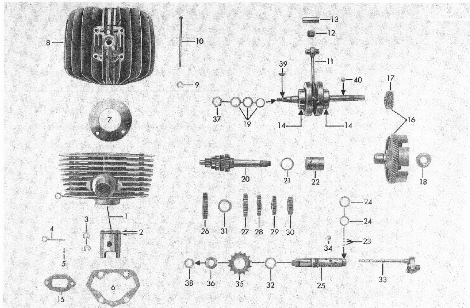
Tafel 15/1 Zylinder, Kurbelwelle, Getriebe Table 15/1 Cylinder, crankshaft, gearbox Planche 15/1 Cylindre, vilebrequin, boîte de vitesses
