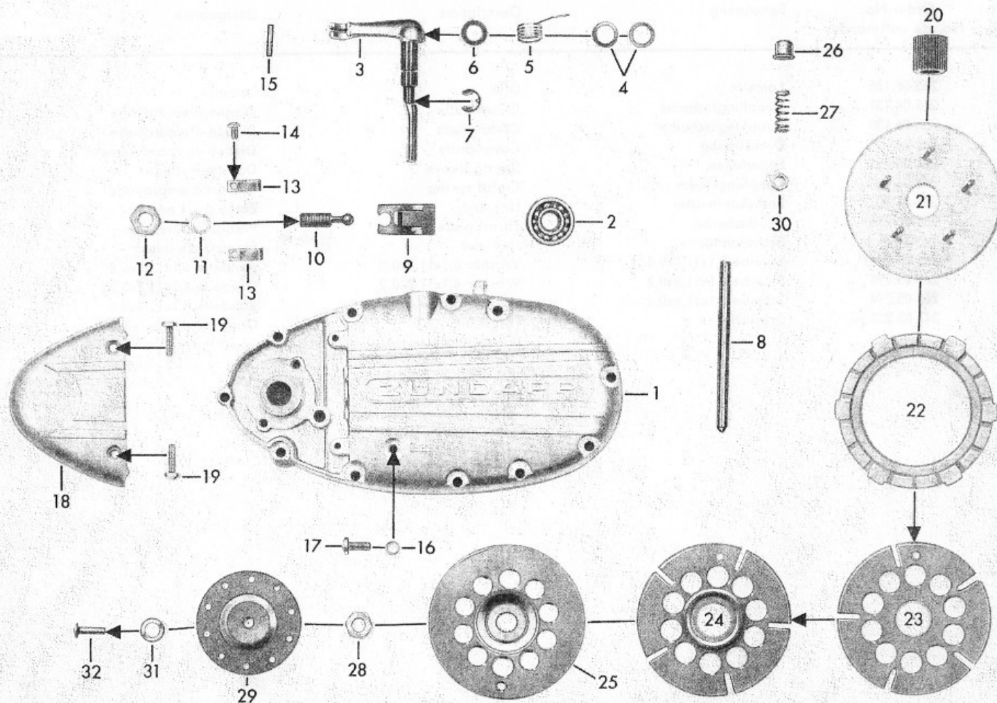
Tafel 14/2 Gehäusedeckel rechts, Kupplung Table 14/2 Casing cover right, clutch Planche 14/2 Couvercle de carter droit, embrayage
