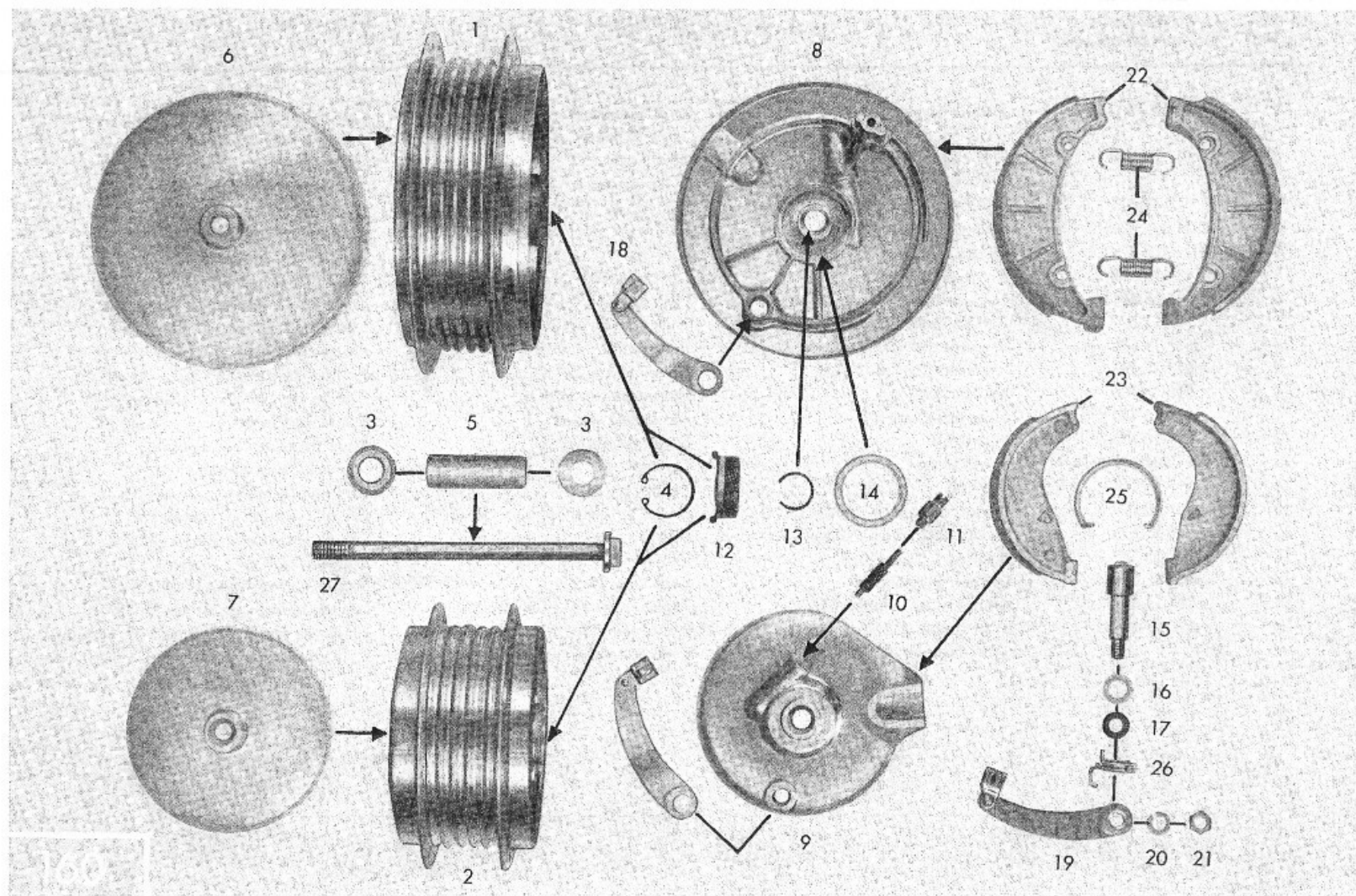
Tafel 23/2 Vorderes Laufrad, Vorderradnabe Table 23/2 Front wheel, front wheel hub Planche 23/2 Roue AV, moyeu de roue AV
