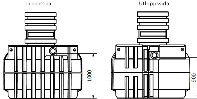
TVÄRSEKTION
