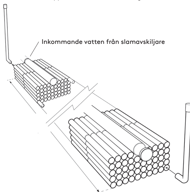
Förminsning vid pumpning PEM 40 Inloppet vrids till sitt översta läge.
