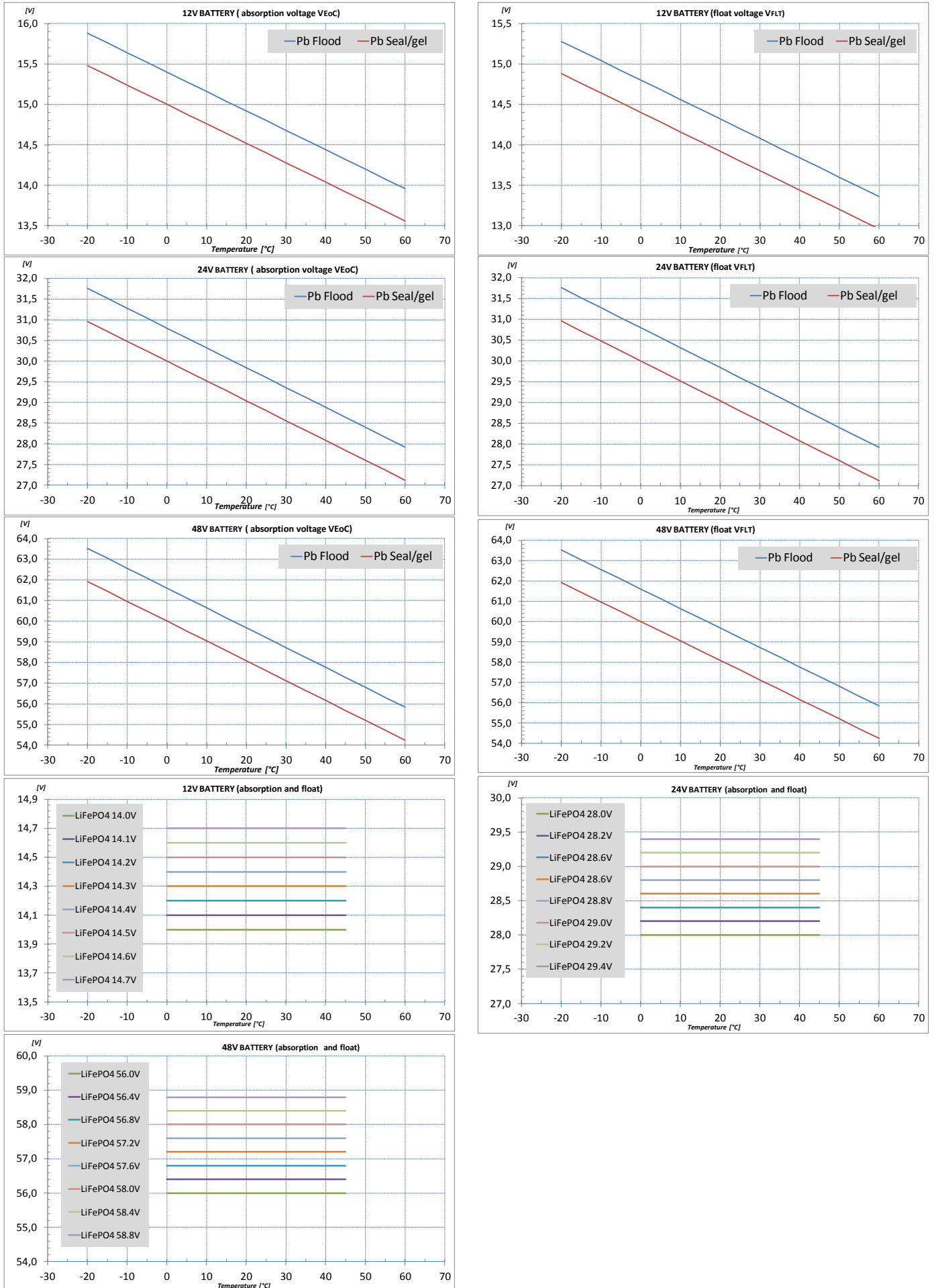
Fig.5 - Absorption voltage e float voltage in funzione della temperatura
