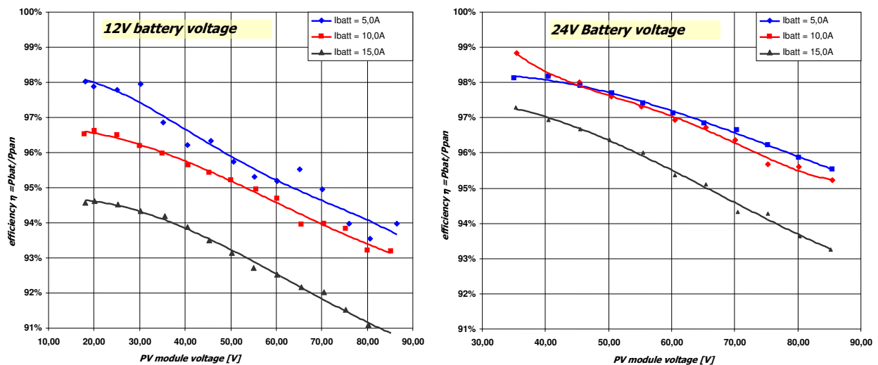
Abb. 7 Leistung des WRM15 dualB/dualB-E je nach Spannung der Solarzelle für das System zu 12 V und 24 V
