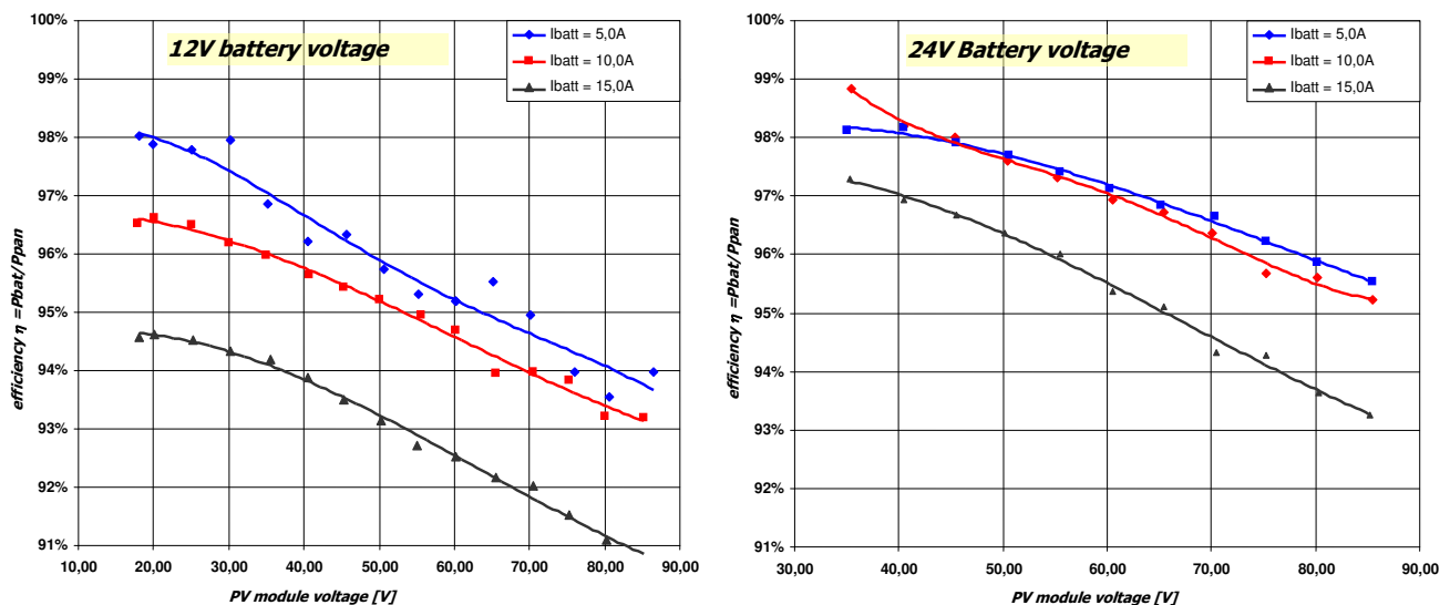
Fig. 7 Rendement du dispositif WRM15 dualB/dualB-E en fonction de la tension du panneau pour un système à 12V et 24V
