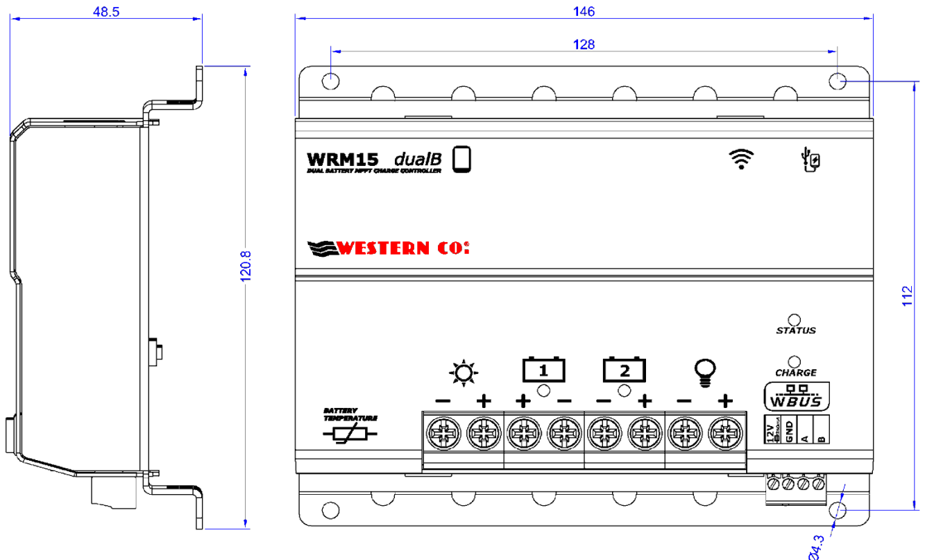
Abb. 5 Ausmaße (mm)
