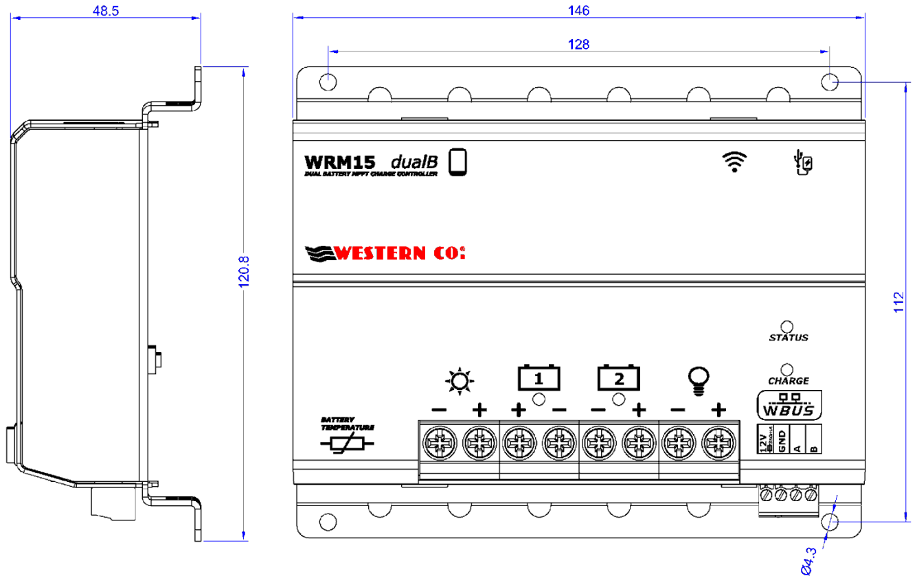
Fig. 5 Dimesions (mm)
