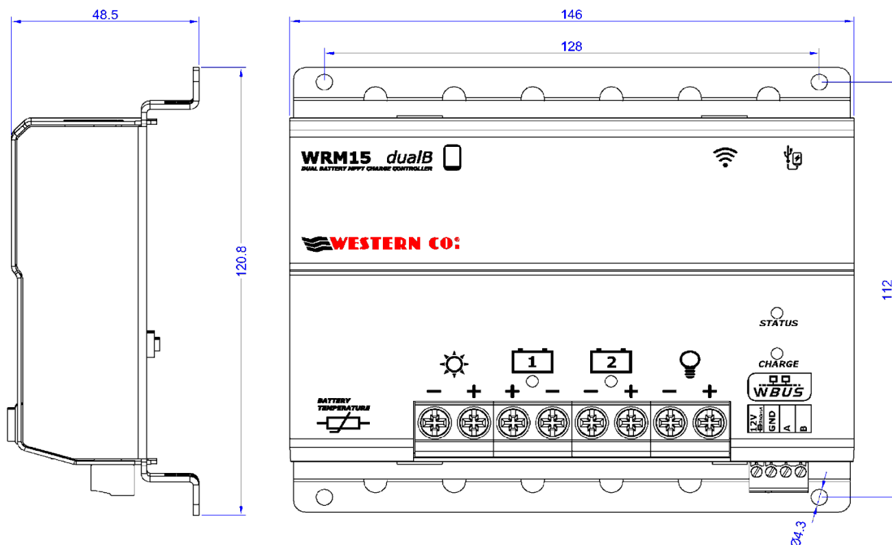
Fig. 5 Dimensioni (mm)
