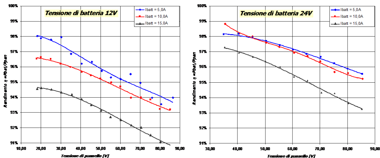
Fig. 7 Rendimento del WRM15 dualB/dualB-E in funzione della tensione di pannello per sistema a 12V e 24V
