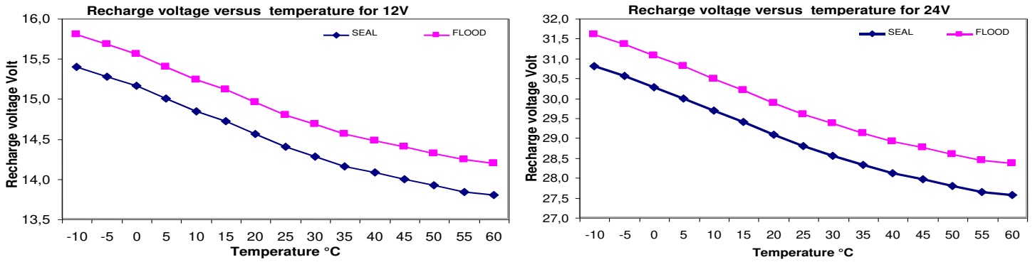
Abb.3 Kompensationskurve der Ladespannung Veoc je nach Temperatur der Batterie
