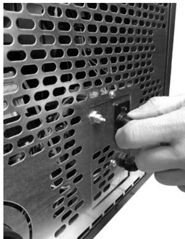
Fig. 34 - Manuell aktivering: MODO AIRTIGHT e QUASIMODO 3 UP
