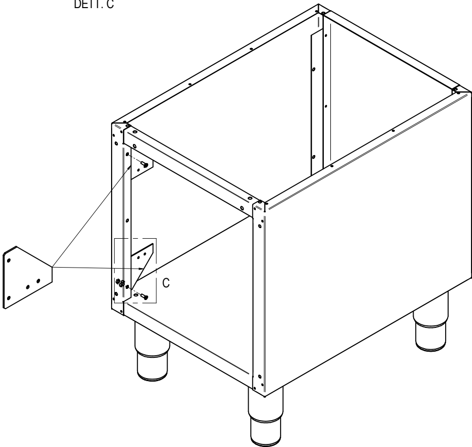
DETT. C
