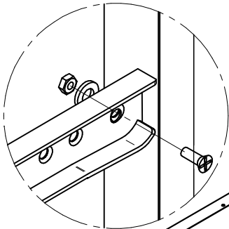
DETT. A
