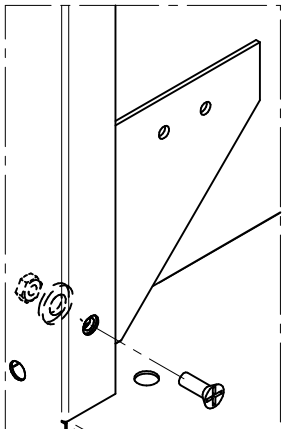
DETT. C
