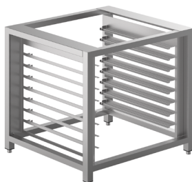
TVL420 Kapacitet 16 plåtar Pelare installation Mått (BxDxH) 800x747x900/950 mm
