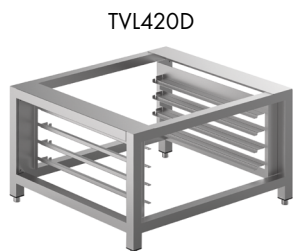
TVL420D Kapacitet 4 plåtar Pelare installation Mått (BxDxH) 800x747x504 mm
