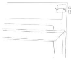
5. Démonter le pivot de la charnière en haut.
