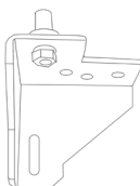
10. Den Stift vom unteren Scharnier wieder auf dem gedrehten Scharnier montieren.
