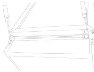
2. Bodenscharnier und Stützbeschlag abmontieren.
