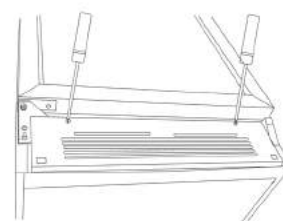
12. Monteer de steunfitting op de tegenoverliggende kant.
