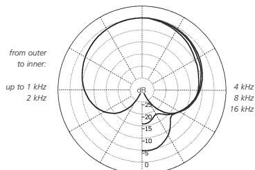
Polar diagram CCM 4VP, CCM 4VXP
