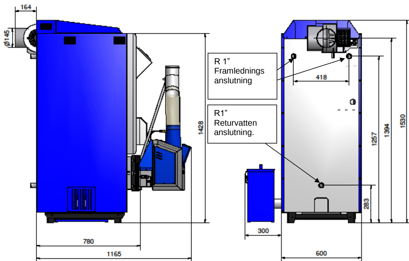
Figur 2 Måttskiss Janfire Pelletspanna
