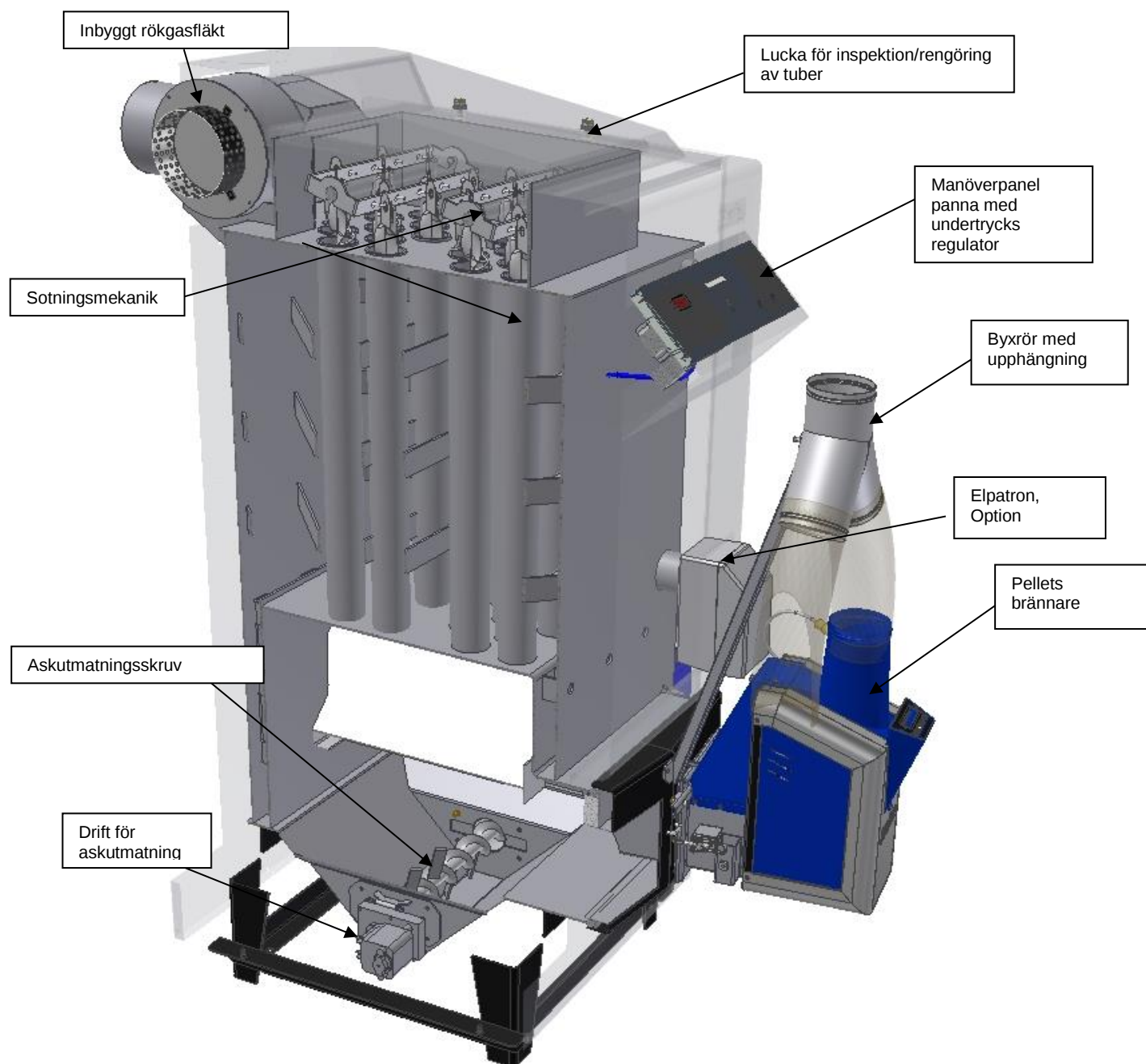
Figur 3 Översiktsbild
