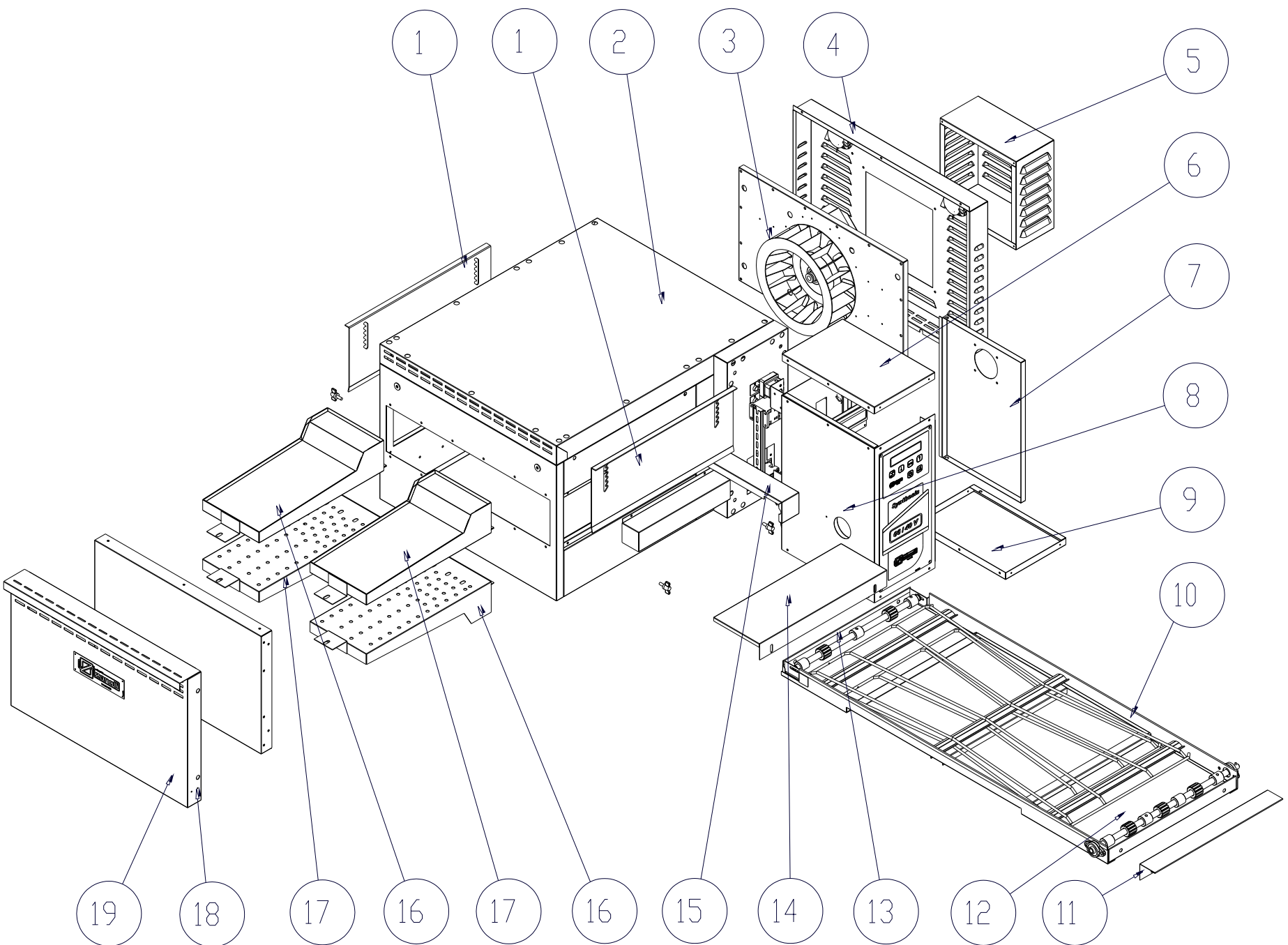
FIG. 10-3 Esploso componenti carpenteria Synthesis 06/40V
