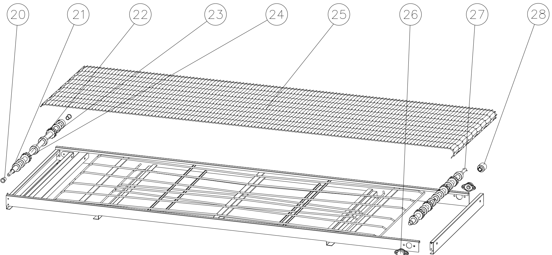
FIG. 10-4 Esploso rete di trascinamento Synthesis 06/40V
