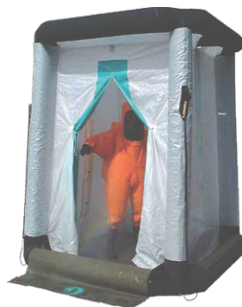
DC200 2,5 x 2,5 x 2,7m 55 kg
