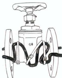
Fig. 2 Lindning av värmekabel runt komponent Se 7 716 260
