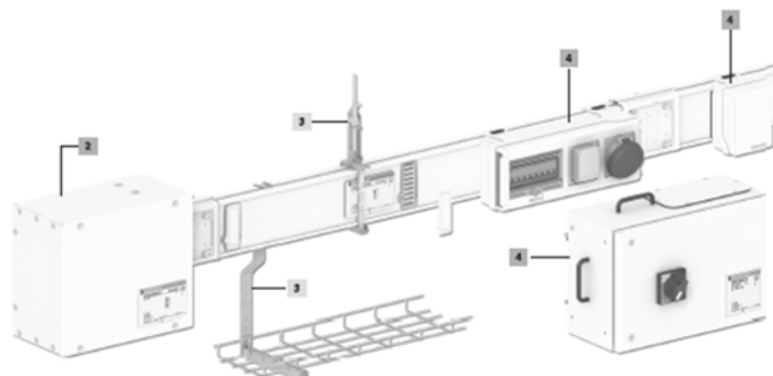
Pendlar för kanalskena
