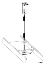
Wirependel
