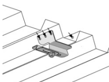
Takfäste för trapetsplåt (stål inkl. borrh., poppnit, självborrh. skruv )
