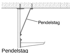
Pendelstag
