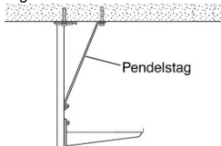
Pendelstag
