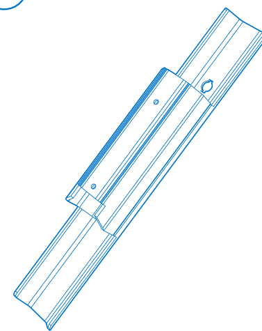
Capot de protection d'angle
