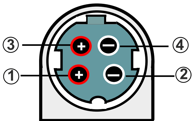
4-Pin typ-E + på pin 1&3
