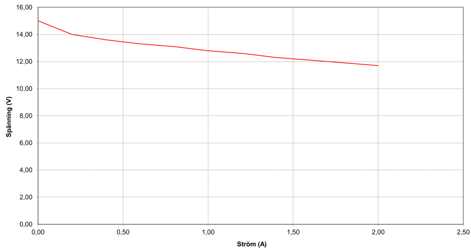
Belastningskaraktistik 8512-0028 230/12 V
