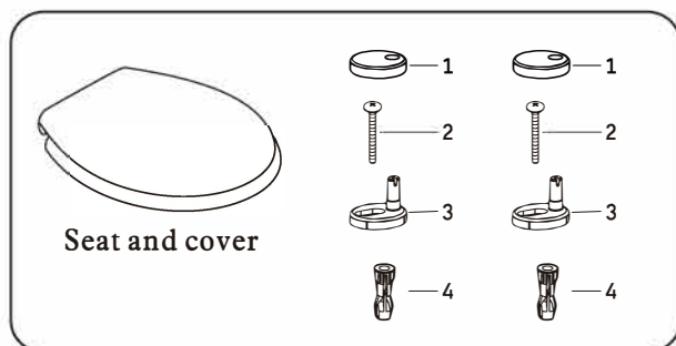
Hinge set.
