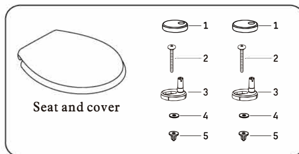
Hinge set.
