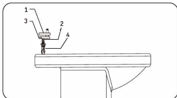
Hinge set.
