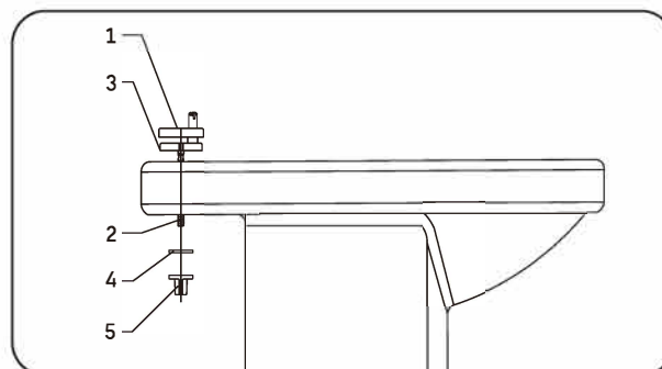
Hinge set.
