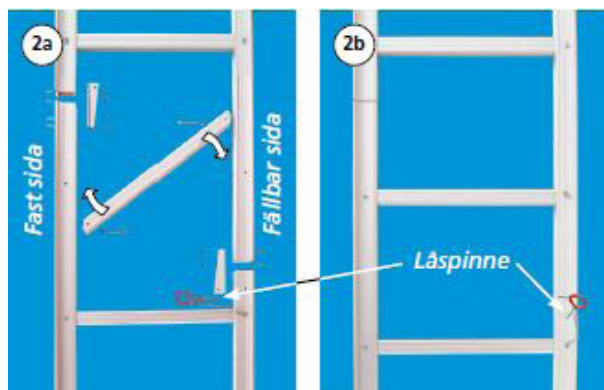
Bilderna 2a och 2b visar öppningsbar skarvning. Skarvsats bestående av 1 st stegpinne, 2 st skarvbeslag med skruv och mutter. Art nr 62-0003.
