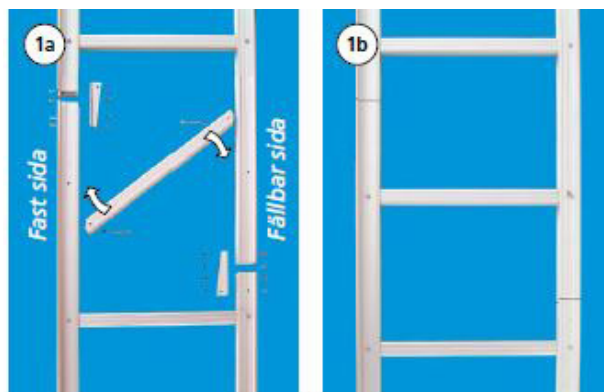
Bilderna 1a och 1b visar fast skarvning. Skarvsats bestående av 1 st stegpinne, 2 st skarvbeslag med skruv och mutter. Art nr 62-0003.
