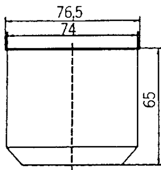
Måttritning
