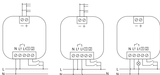
Koppling för 0-10 V bus (utan brytning av matning till last)
