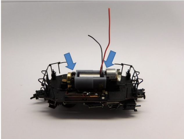
Stifte platzieren Mount pins Plaats de pinnen
