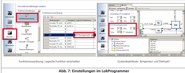
Abb. 7: Einstellungen im LokProgrammer
