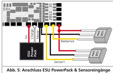
Abb. 5: Anschluss ESU PowerPack & Sensoreingänge
