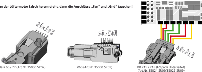
Abb. 6: Anschluss Raucheinheiten
