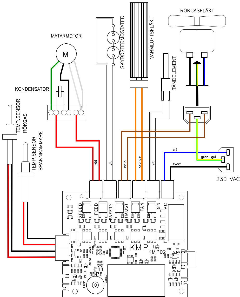
Kopplingsschema
