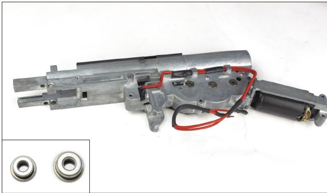
6mm & 8mm軸承比較
