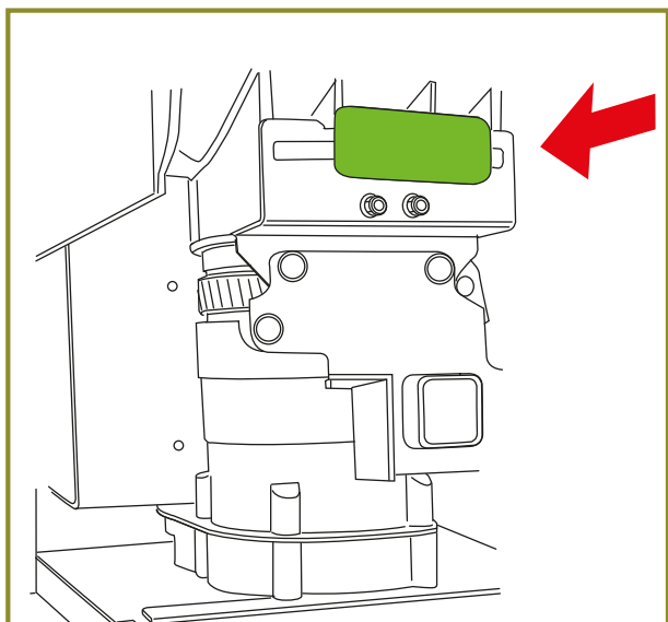
6. Tryck in den eller de gröna slutaren/slutarna med ett kraftfullt tryck, rakt in tills det tar helt stopp.
