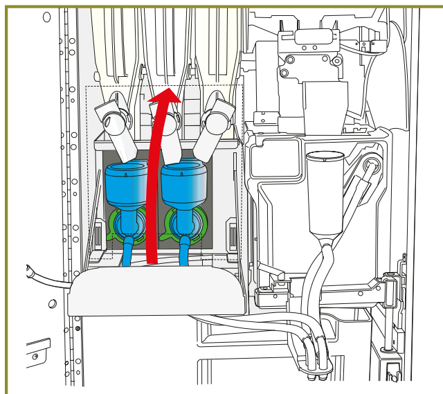
15. Vik upp luckan framför produktbehållarna.
