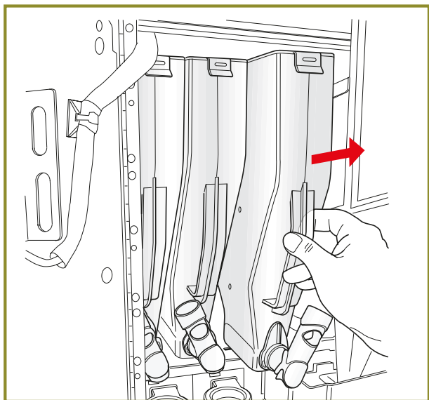
4. Lyft ur produktbehållarna och ställ dem på bänken.
