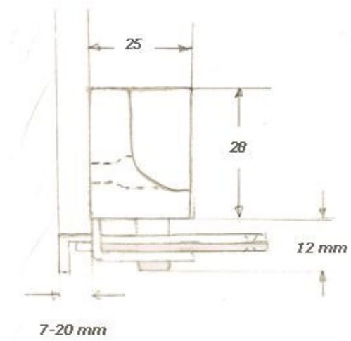
Måttskiss fönsterlås 750-Inåtgående
