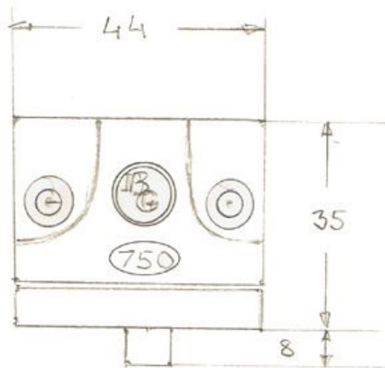
Måttskiss fönsterlås 750-Utgående
